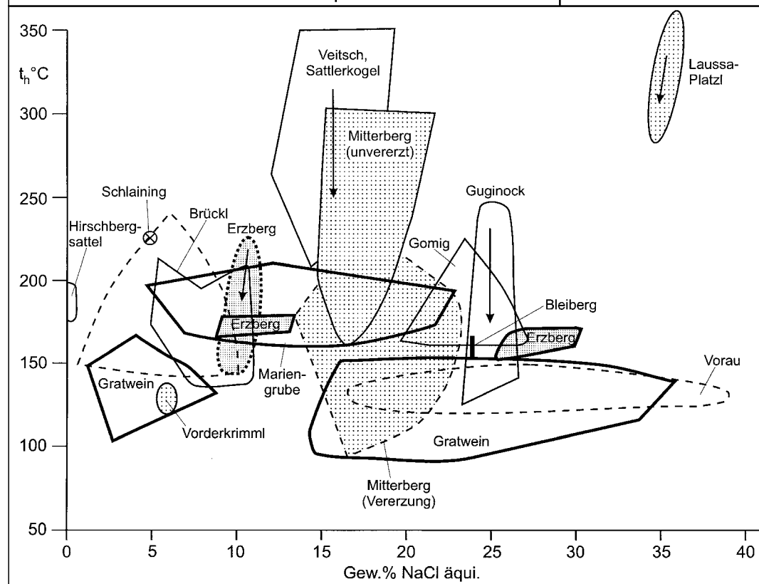
Abb. 390. a) Diagramm (oben) T_h vs. Gew.-% \text{NaCl}_{\text{äquiv.}} mit den Daten der Scheelitlagerstätte Fel- bertal und der Magne- sit-(Scheelit-)lagerstät- te Tux-Lanersbach. b) Diagramm (unten) T_h vs. Gew.-% \text{NaCl}_{\text{äquiv.}} mit Daten anderer ost- alpiner Mineralisatio- nen.
