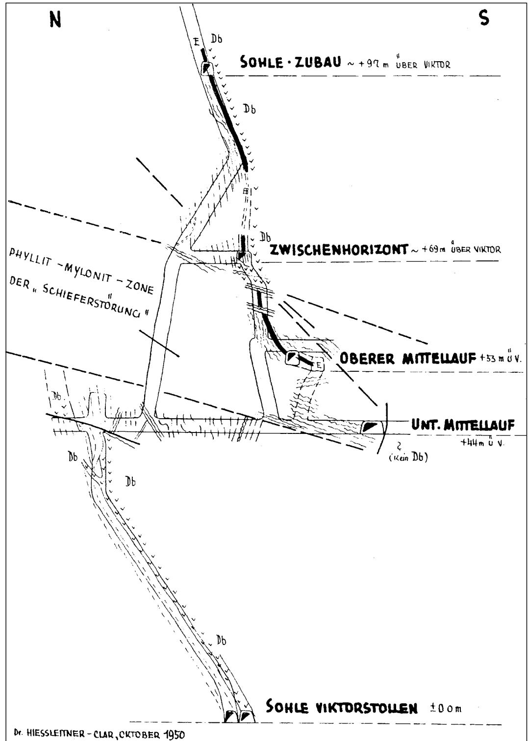
Abb. 259. N-S-Saigerschnitt durch die Pb-Zn-Lagerstätte von Tösens in der Ebene des Querschlaßes am unteren Mittellauf mit der Aufbruchverbindung vom Viktor- zum Zubaustollen. Nach HIESSLEITNER, G. & CLAR, E. (1950).
