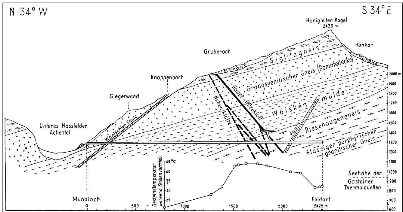
Abb. 247. Profil längs der Stollenachse des Radhausberg-Unterbaues mit Eintragung der von K. ZSCHÖCKE gemessenen Gesteinstemperaturen während des Stollenvortriebs. AUS EXNER, C. (1950).
