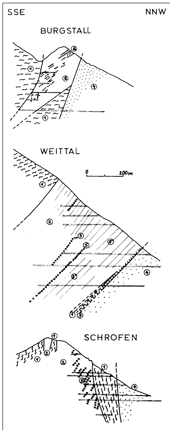
Abb. 277. Profile durch die Lagerstätten des Fahlerzbezirkes Schwaz – Brixlegg. 1 = paläozoischer Phyllit; 2 = Devondolomit; 3 = Untertriadische Basalbreccie; 4 = Buntsandstein; 5 = Fahlerzvererzung. Aus VOHRZYKA, K. (1968), nach PIRKL, H. (1961).
