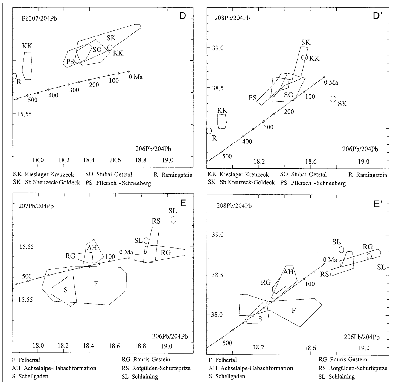
Abb. 375. Bleiisotope in Erzen ostalpiner Lagerstätten.
