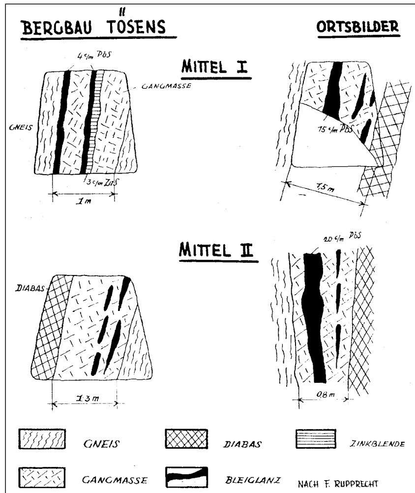
Abb. 260. Ortsbilder aus der Pb-Zn-Lagerstätte Tösens. Nach F. RUPPRECHT, aus HIESSLEITNER, G. & CLAR, E. (1950).
