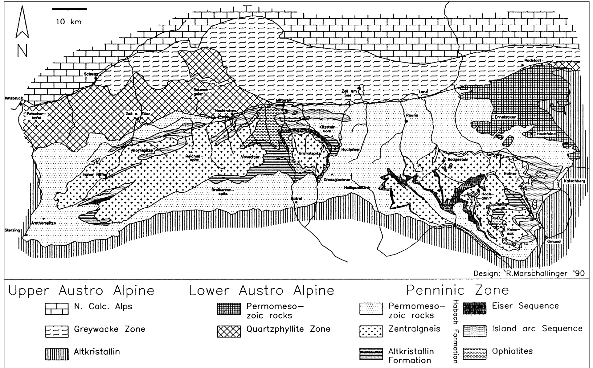
Abb. 70. Prä-permomesozoische Schichtenentwicklungen und Gliederungen der Habach-Gruppe im Tauernfenster. Aus Höck, V. (1993).
