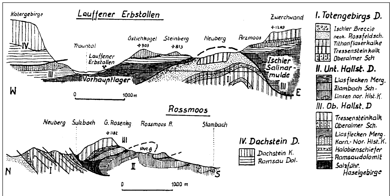
Abb. 314. Salzagerstätte Bad Ischl: Profile durch den Lauffener Erbstollen. Nach MEDWENITSCH, W. (1958).
