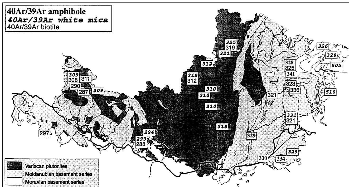
Abb. 16. Variszische Abkühlalter in der südöstlichen Böhmisches Masse. Aus KLÖTZLI, U. et al. (1997).
