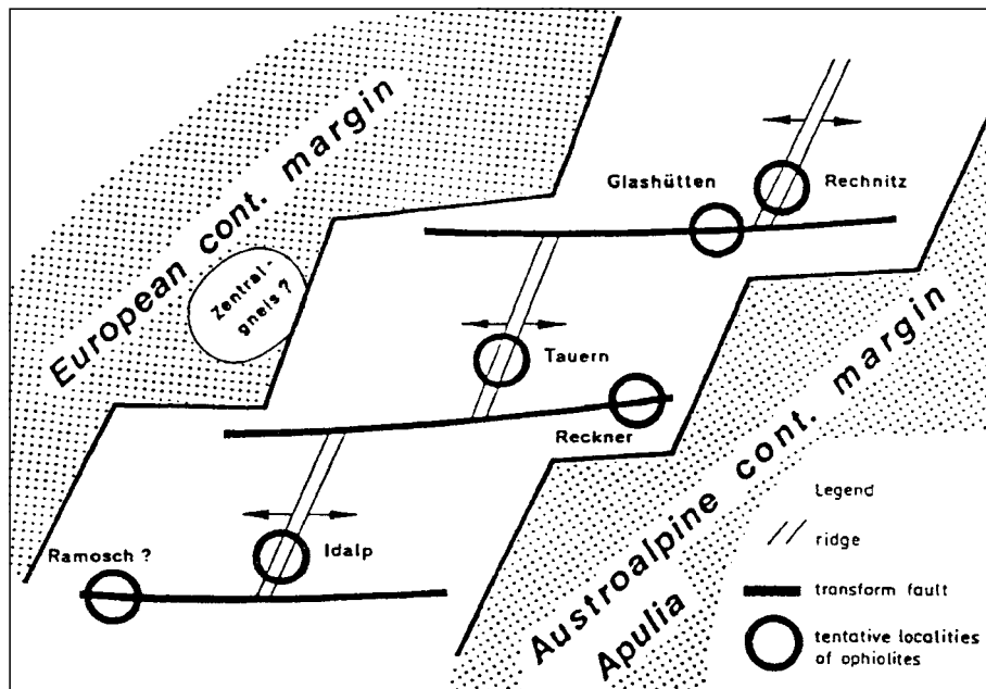
Abb. 67. Bildungspositionen von Ophiolithen in den Ostalpen im Engadiner Fenster (Ramosch, Idalp), des Reckners (Tarntaler Alpen), der Hohen Tauern und der Rechnitzer Serie. Aus KOLLER, F. & HÖCK, V. (1992).
