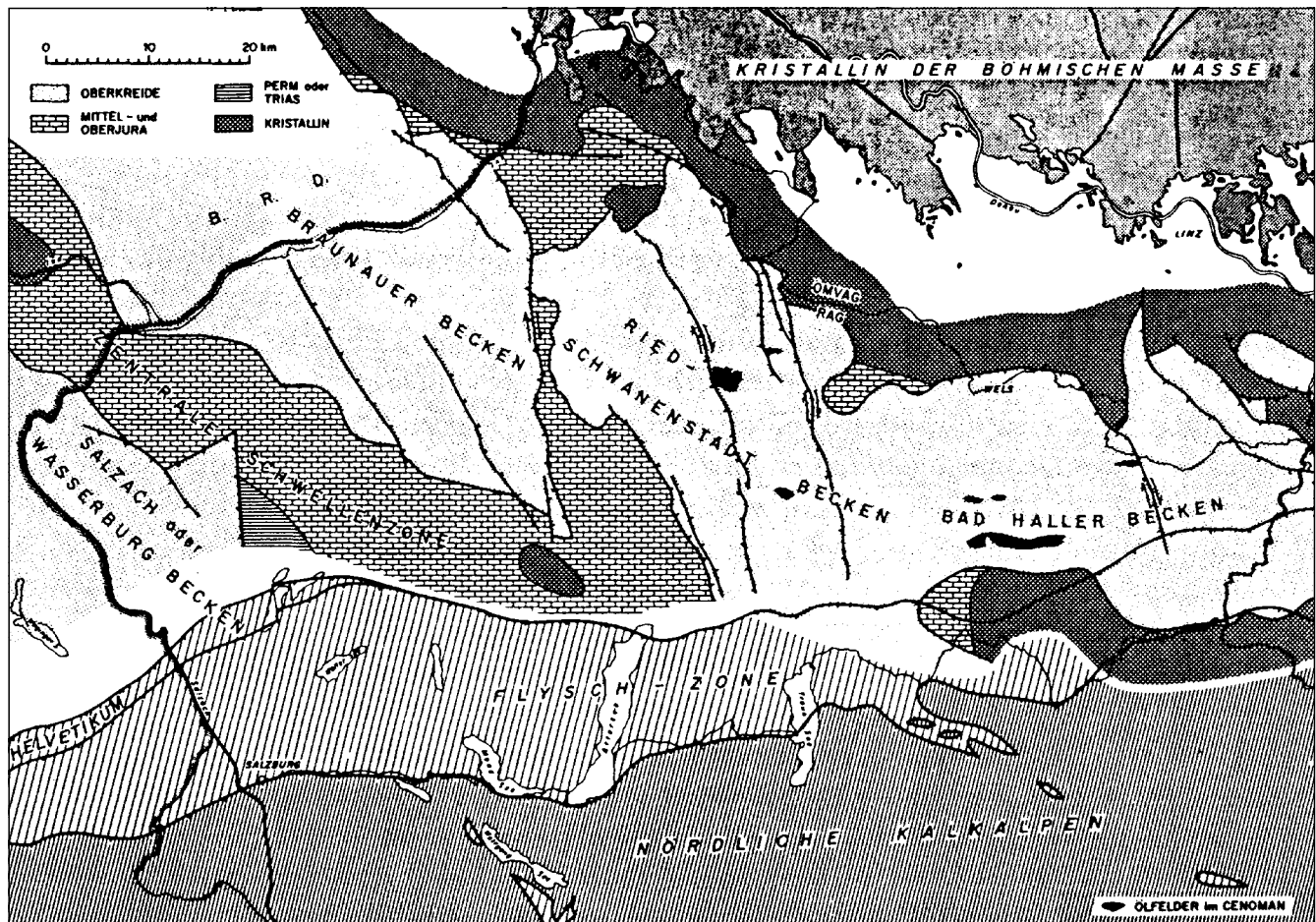
Abb. 25. Der Molasseuntergrund zwischen Inn und Enns. Nach WEBER, F. et al. in WAGNER, L. (1980).
