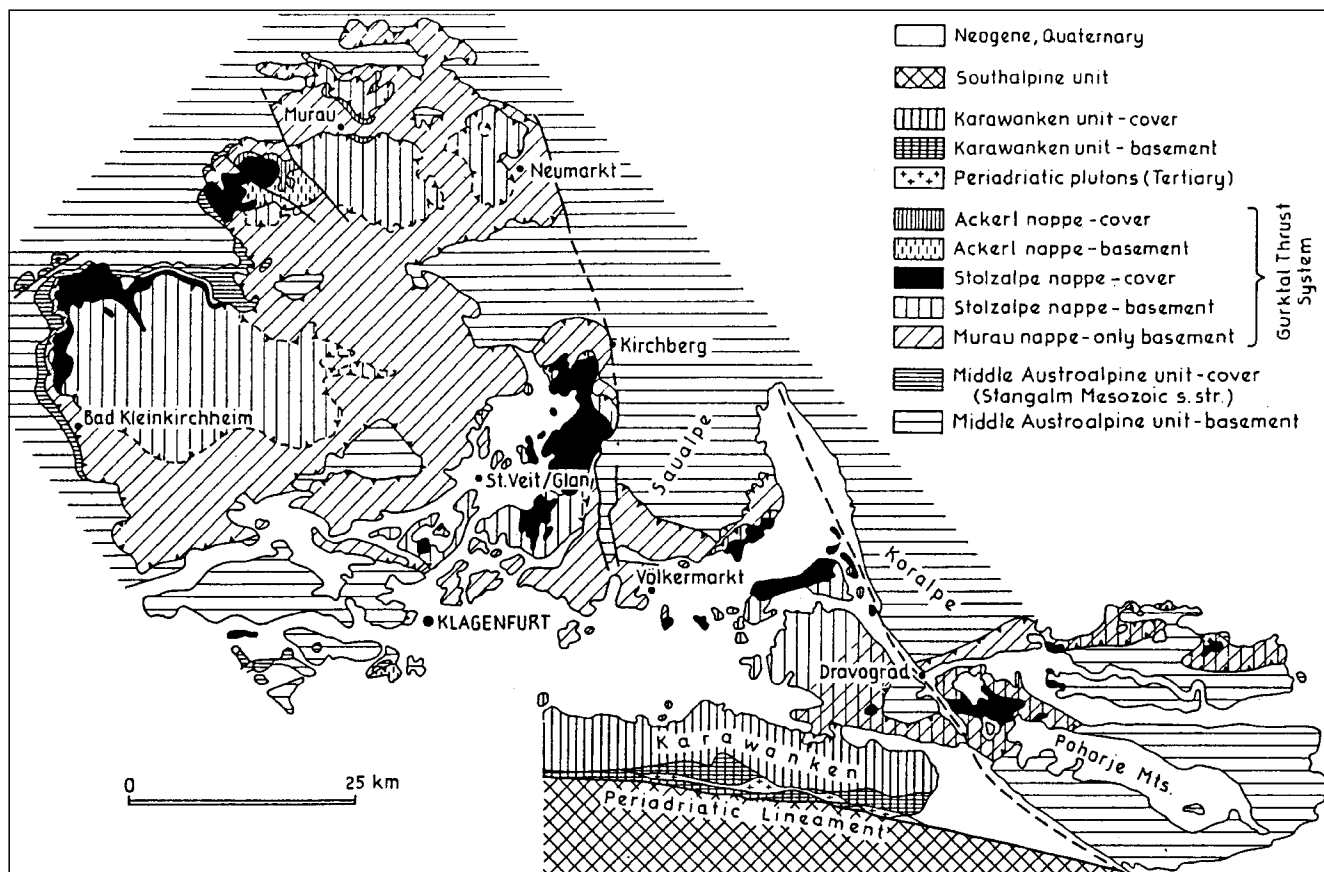
Abb. 160. Tektonische Gliederung des Gurktaler Deckensystems. Aus NEUBAUER, F. (1987).
