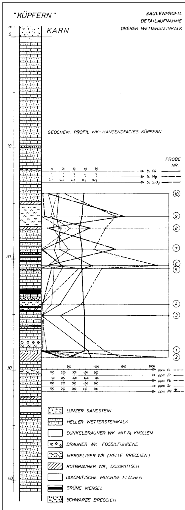
Abb. 311. Schematisches Profil durch das Blei-Zink-Vorkommen von Kuppern (Oberösterreich). Aus WERNECK, W. (1974).
