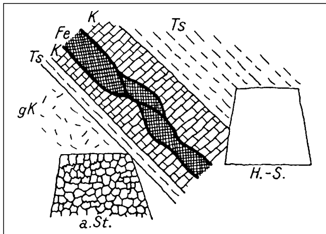
Abb. 287. Geologisches Profil durch die Sideritlagerstätte der Hocheckbaue (Eyweggsattel; Ulmenbild Tatzlstollen). H.-S. = Hauptschlag; a. St. = alte Strecke. Ts = grauer Phyllit; K = grauer Kalk; Fe = Spateisenstein; schwarze, kräftige Linien = Thuringitschiefer. Nach CLAR, E., aus REDLICH, K.A. (1931).
