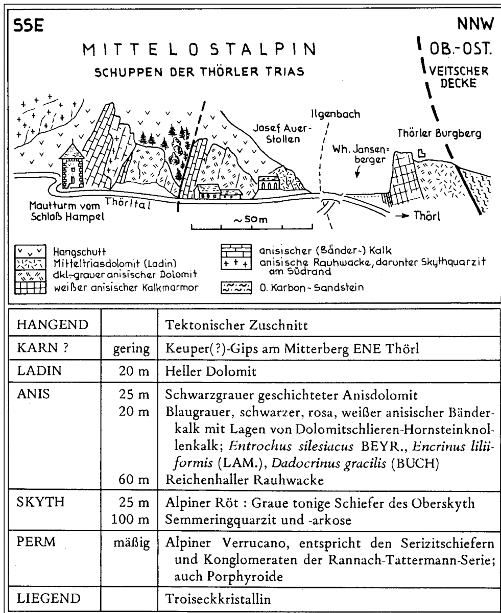
Abb. 129. Schichtfolge und Profil durch das zentralalpine Mesozoikum bei Thörl. Aus TOLLMANN, A. (1977a).
