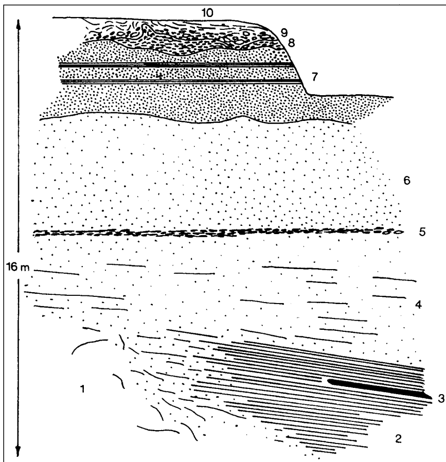
Abb. 218. Profil durch die kohleführenden Melker Schichten in einem Sandgrubenaufschluß S Oberwölbling. 1 = kaolinisierter Granulit; 2 = Pielacher Tegel; 3 = Kohlenflöz; 4 = tonig-sandige Vertreter des Pielacher Tegels; 5 = Granulitgeröllhorizont; 6 = Älterer Melker Sand; 7 = Jüngerer Melker Sand mit Tonzwischenlagen; 8 = Hollenburg-Karlstettener Konglomerat; 9 = Schotter der Köbling-Flur; mit 8 frostgestaucht; 10 = Solifluktionsschutt. Aus UCHS; (1972b).
