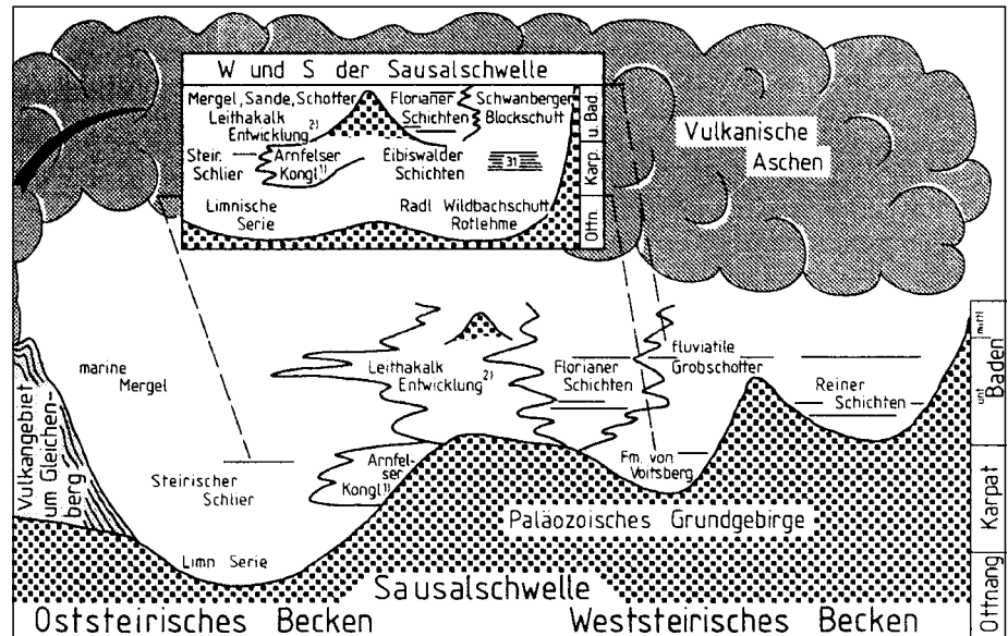
Abb. 227. Schematische Darstellung der Tuff führenden Schichten im Miozän des Ost- und Weststeirischen Tertiärbeckens. Aus EBNER, F. & GRÄF, W. (1982).
