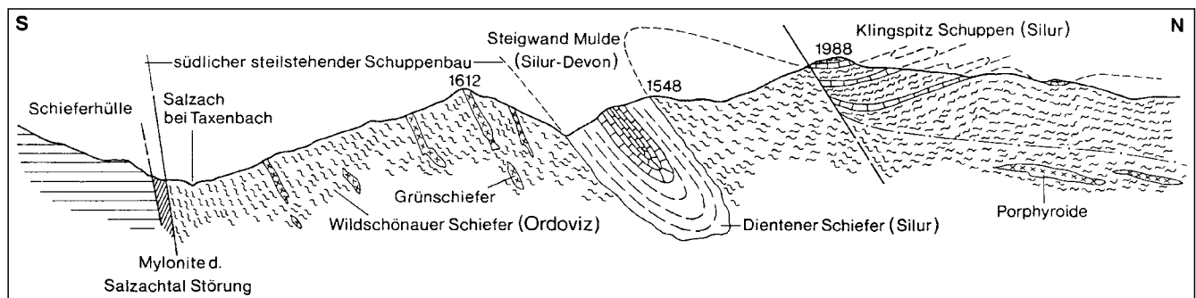
Abb. 147. N-S-Profil durch die Salzburger Grauwackenzone südlich von Dienten. Aus BAUER, F.K. et al. (1969).
