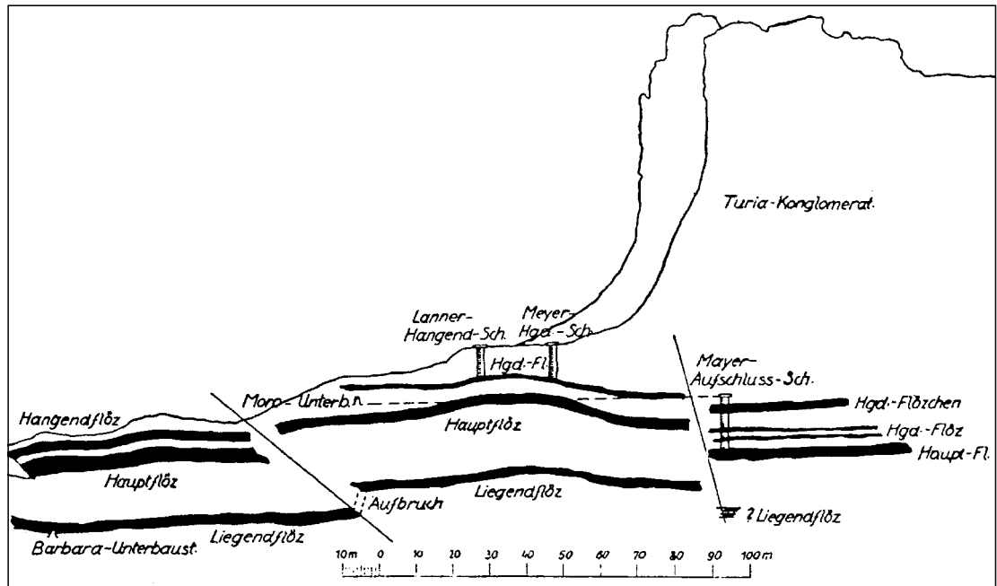
Abb. 233. Profil durch die Braunkohlenvor- kommen des Tu- riawaldes. Aus PETRASCHECK, W. (1922/25).
