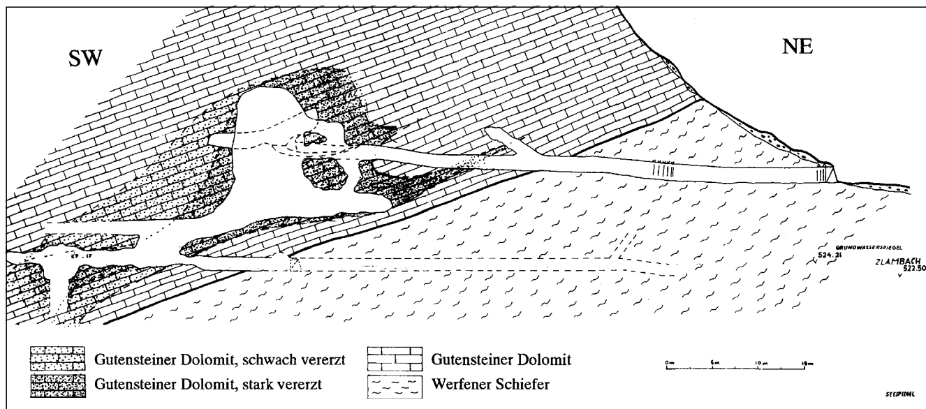
Abb. 310. Profil durch das Pb-Zn-Vorkommen Arikogel am Hallstätter See. Aus HASLINGER, E. (1962).
