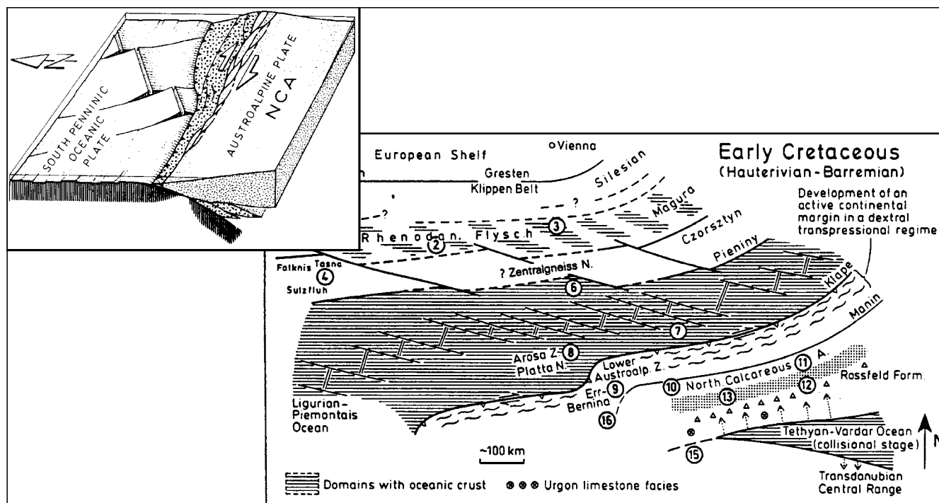
Abb. 97. ▼▼▼ a) Modell der tektonischen Erosion von Teilen der Kalkalpen im Campan/Maastricht durch die schräg verlaufende penninische Subduktion. Aus WAGREICH, M. (1995). b) Paläogeographische Position des Ostalpins in der Unterkreide. Nach FAUPL, P. & WAGREICH, M. (1992). c) Plattentektonisches Modell für die Oberkreide der Ostalpen. Aus WAGREICH, M. & FAUPL, P. (1994b).
