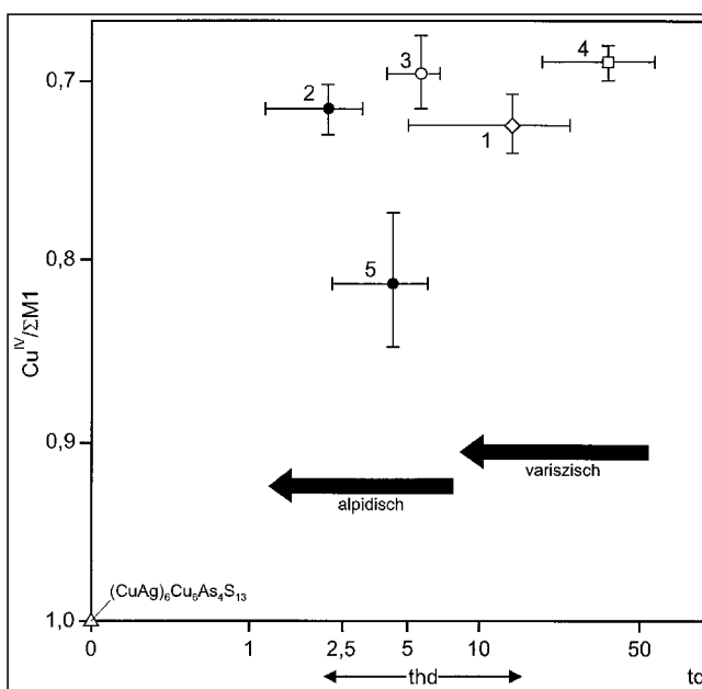
Abb. 343. Varianz der chemischen Zusammensetzung der Fahlerze von Leogang. Die mineralparagenetisch vorgegebenen Gruppierungen sind mit Mittelwert und Standardabweichungen dargestellt. Balkenlänge entspricht der Standardabweichung! 1 = PbS-Paragenese (syndementär), Schwarzleo; 2 = Fahlerzkluft (junge Mineralisation), Schwarzleo; 3 = Hg-Ag-Paragenese (jüngste Mineralisation), Schwarzleo; 4 = Gersdorffit-Paragenese (Nöckelberg); 5 = Bornit-Paragenese (Nöckelberg). Nach LENGAUER, C.L. (1988).
