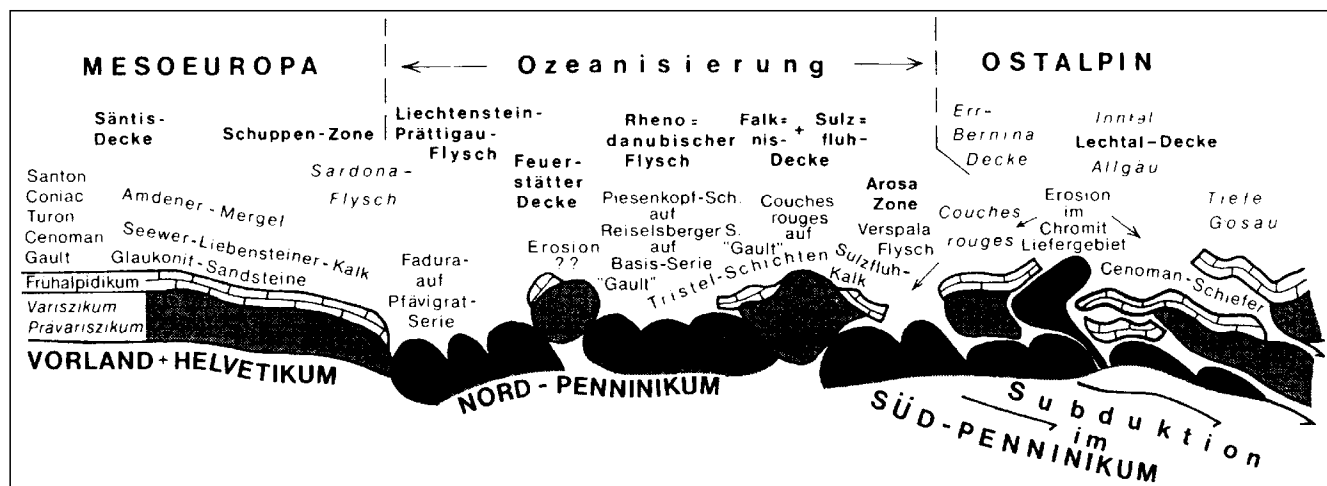
Abb. 58. Primäre Position des Rhenodanubischen Flyschs und der Feuerstätter-(Wildflysch-)Decke im Nordpenninikum (OBERHAUSER, R., 1980b).
