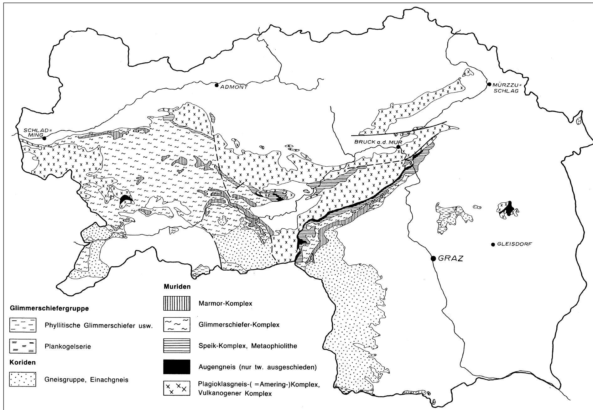
Abb. 125. Die lithologische Gliederung des „mittelostalpinen“ Kristallins in der Steiermark (aus FLÜGEL, H.W. & NEUBAUER, F., 1984). In der metallogenetischen Karte wird das Schladminger Kristallin dem Unterostalpin angegliedert.
