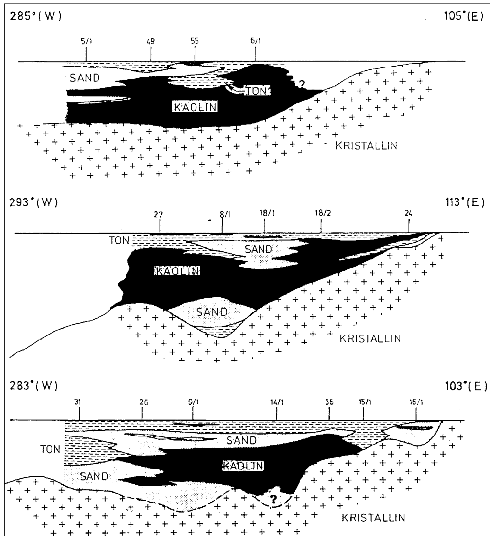
Abb. 212. Geologische Profile durch die Kaolinlagerstätte Niederfladnitz bei Retz, Waldviertel, N.Ö. Nach AUSTROMINERAL (1978).
