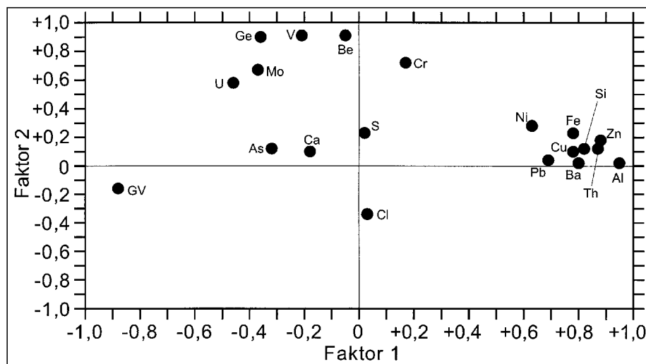
Abb. 355. Hauptkomponentenanalyse chemischer Daten österreichischer Braunkohlen. Faktor 1 vs Faktor 2 (GV Glühverlust). Es wird eine Gliederung in drei Element- gruppen erkennbar: vornehmlich an die Tonsubstanz gebundene Elemente (Clu- ster mit Al und Si), stärker an die organi- sche Substanz gebundene Spurenelemen- te (As, U, Mo, V, Ge, ?Be, ?Cr) und Eleme- nte ohne signifikante Beziehungen (S, Cl). Nach AUGUSTIN-GYURITS, K. & SCHROLL, E. (1992).
