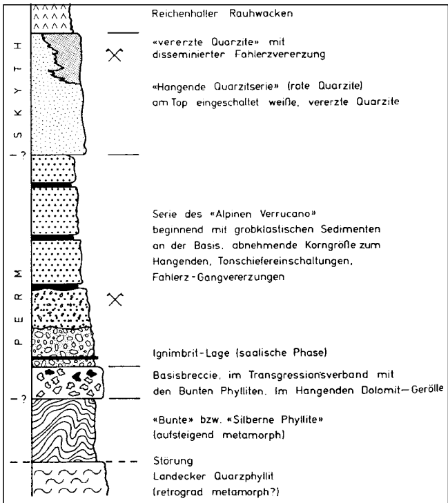
Abb. 305. Schematisches Profil durch die erzführende Quarzitserie im Rammlestobel. AUS HADITSCH, J.G. & KRAINER, K. (1993).
