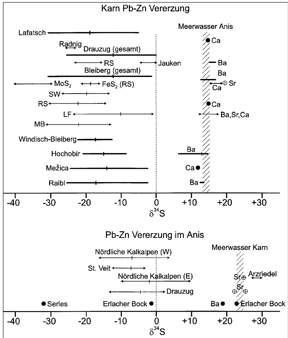
Abb. 368. Sulfat- und Sulfidschwefelverteilung in anisichen und karnischen Pb-Zn-Vererzungen der ostalpinen Trias. SW = Schwellenfazies; RS = Raibler Schiefer (Carditavererzungen); LF = Lagunenfazies (Erzkalkvererzung); MB = Maxer Bänke; Ba = Baryt; Sr = Coelestin; Ca = Anhydrit; Gips; W = West, E = Ost.
