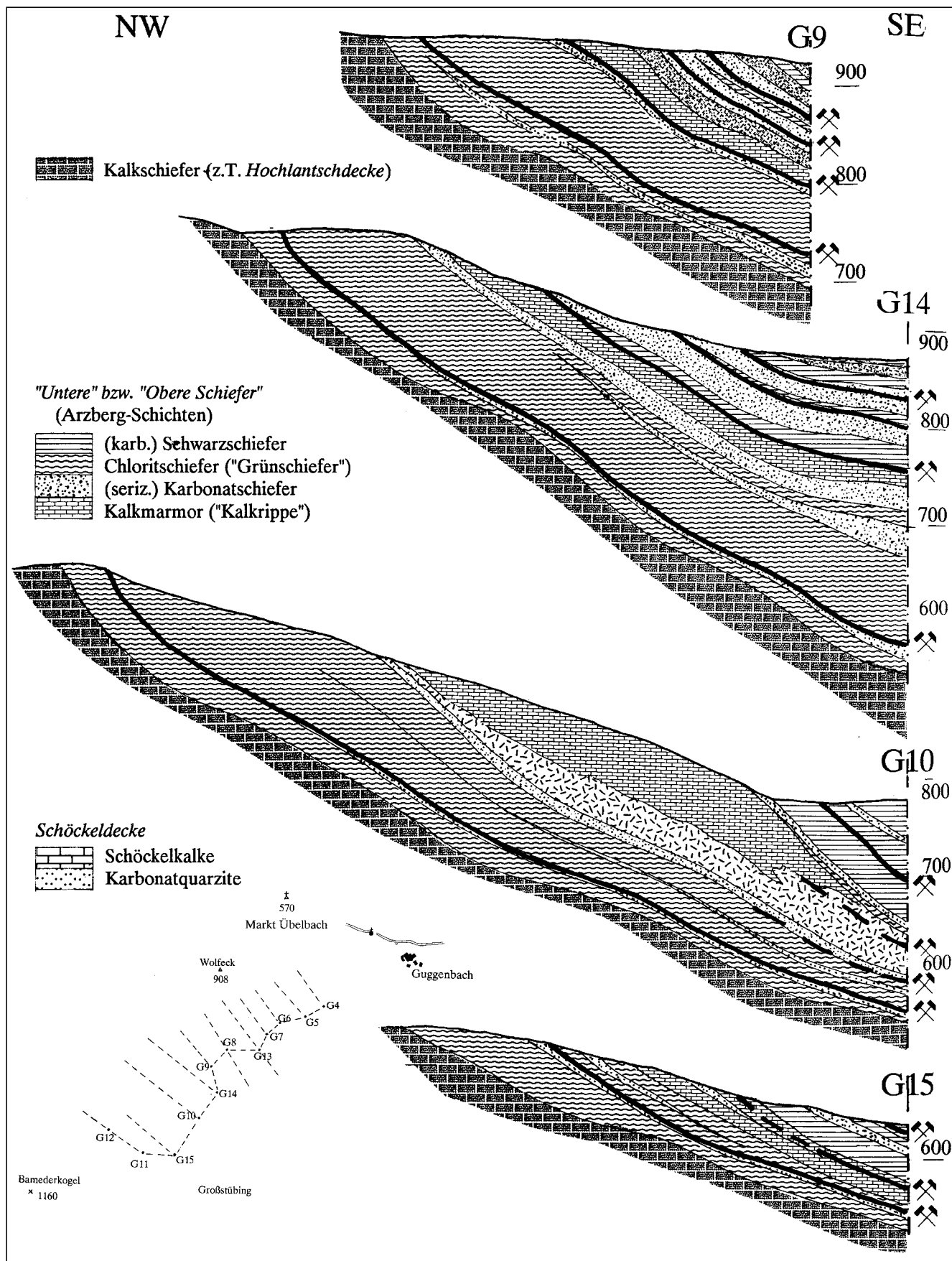
Abb. 290. Querprofile durch die Bohrungen Guggenbach G9, G14, G10 und G15. AUS WEBER, L. (1990).
