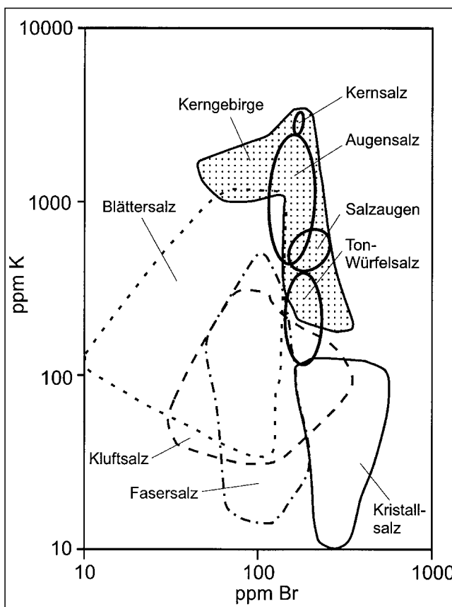
Abb. 352. K/Br-Diagramm primärer und sekundärer Halite. Nach REINOLD, P. (1965).
