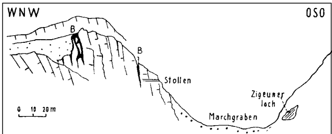
Abb. 333. Profil durch das Bauxitvorkommen am Großen Auriegel. AUS PLÖCHINGER, B., 1961).
