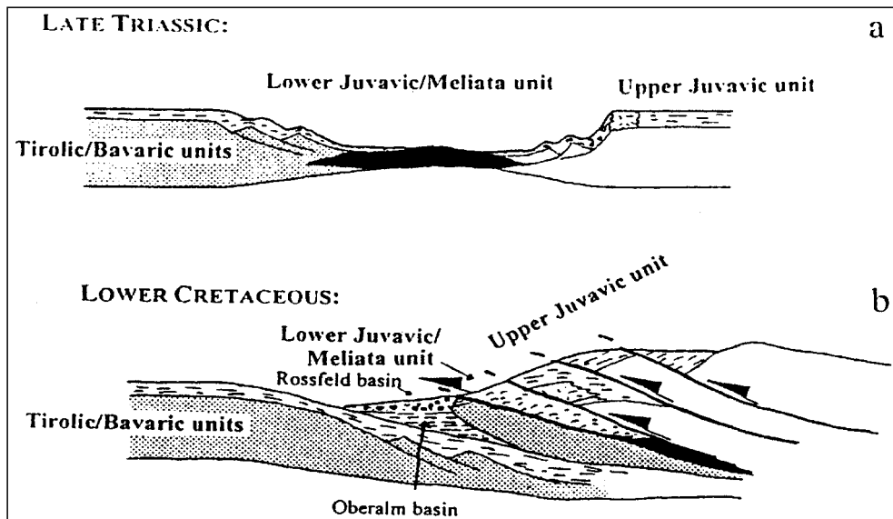
Abb. 96. ►►► Modell der triadischen und unterkretazischen Paläogeographie der Kalkalpen. Aus NEUBAUER, F. & SCHWEIGL, J. (1996).
