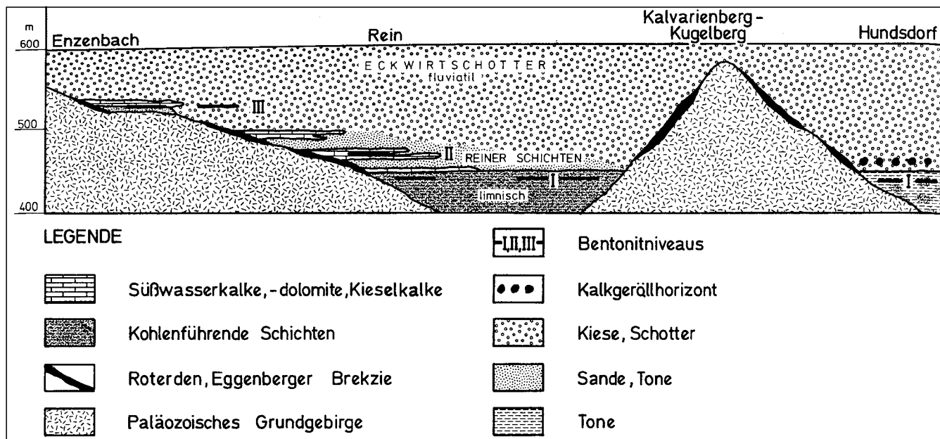
Abb. 230. Schematisches Profil durch das Reiner Becken. AUS EBNER, F. & GRÄF, W. (1982).
