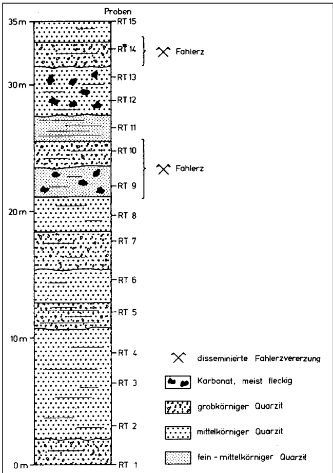
Abb. 304. Schematisches Profil durch die erzführende Permoskythserie im Stanzertal/Arlberg. AUS HADITSCH, J.G. & KRAINER, K. (1993).
