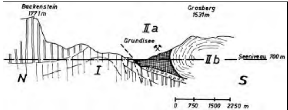
Abb. 318. ►►► Geologisches Profil durch die Gipslagerstätte Wiern/Grundlsee.
