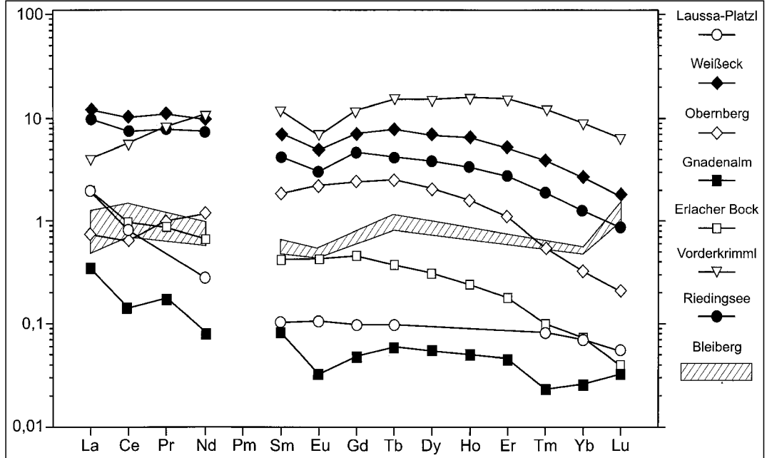
Abb. 347. Chondritnormierte SEE- Verteilung von Fluoriten aus dem Anis und der zen- tralalpiner Trias. ICP-MS- bzw. INAA-Daten im Vergleich mit Fluoriten aus Bleiberg (Mittelwerte der I., II. und III. Genera- tion, INAA, Tab. 9b). Nach GÖTZINGER, M.A., KOSS, S. & SPINDLER, P. (unpubl.)
