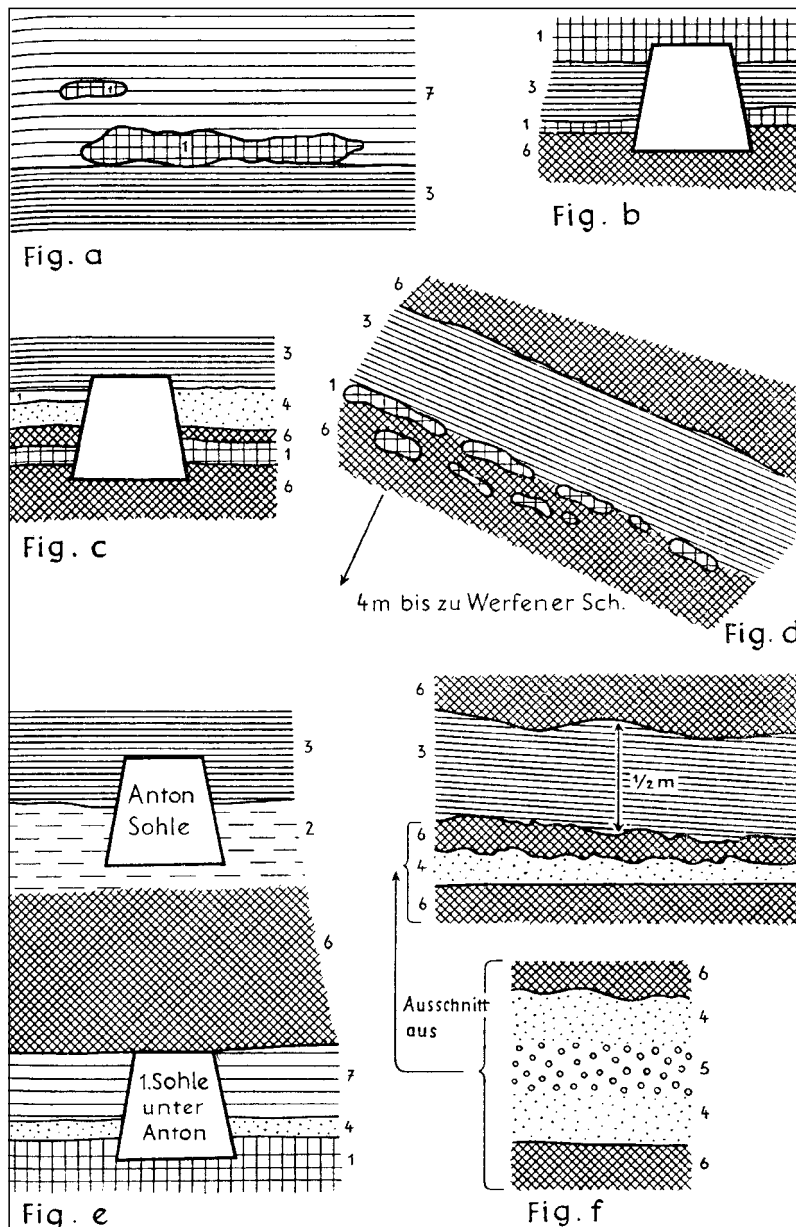
Abb. 301. Ortsbilder aus den Eisenerzlagerstätten von Sulzau – Werfen. 1 = Gutensteiner Dolomit; 2 = Gutensteiner Dolomit (dünn geschichtet); 3 = grüner Mock; 4 = grauer Mock; 5 = Dolomitbreccie; 6 = Brauneisenerz (massig); 7 = Brauneisenerz (geschichtet). Nach HEISSEL, W. (1955).
