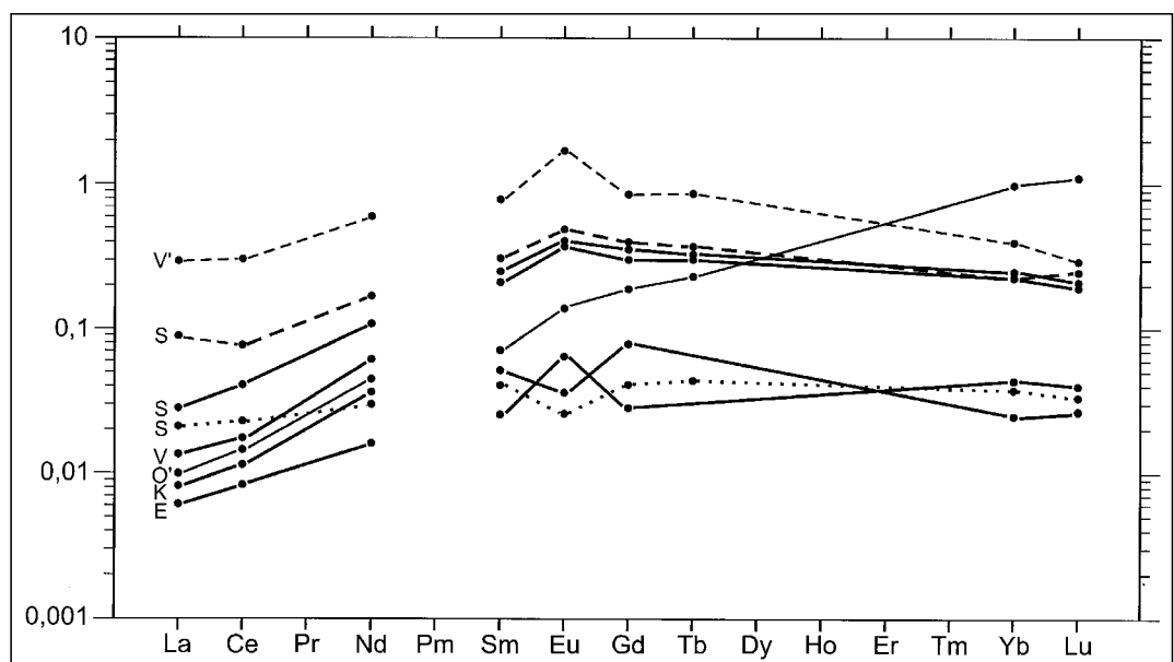
Abb. 349. Beispiele von PAAS-normierten SEE-Mustern von Magnesiten. V = Veitsch; S = Sunk; O = Oberdorf; K = Krauthaus; E = Eichberg.
