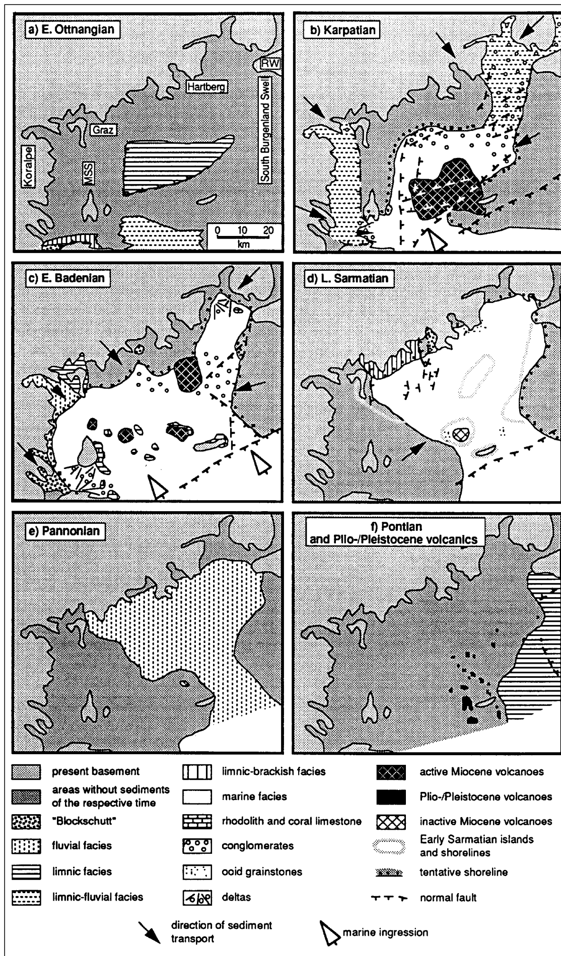
Abb. 42. Paläogeographische Karten des Steiri- schen Beckens. MSS = Mittelsteiri- sche Schwelle; RW = Rechnitzer Fen- ster; Kreuze markie- ren stabile oder He- bungs-Bereiche. Aus EBNER, F. & SACHSENHOFER, R.F. (1995).
