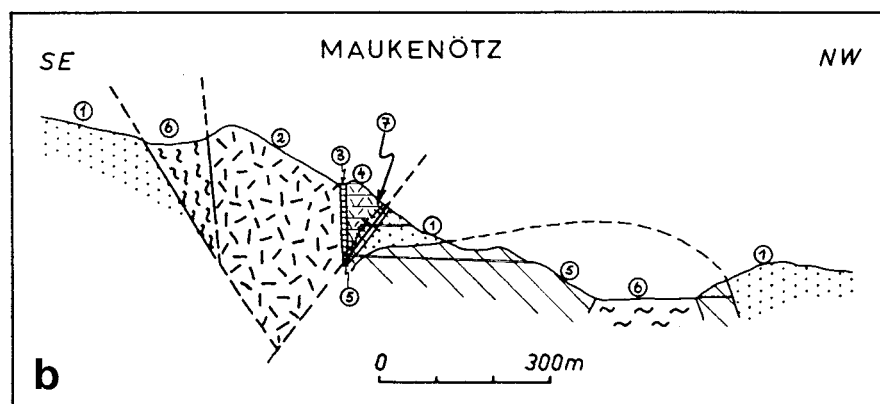
Profil durch die Lagerstätte Maukenözt, vereinfacht, nach H. PIRKL (1961). 1 = Buntsandstein und Werfener Schichten, 2 = Ramsau-Dolomit, 3 = Raibler Schichten, 4 = Dolomit (karn.-nor.), 5 = Devon. Dolomit, 6 = Paläoz. Phyllite, 7 = Fahlerzvererzung.
