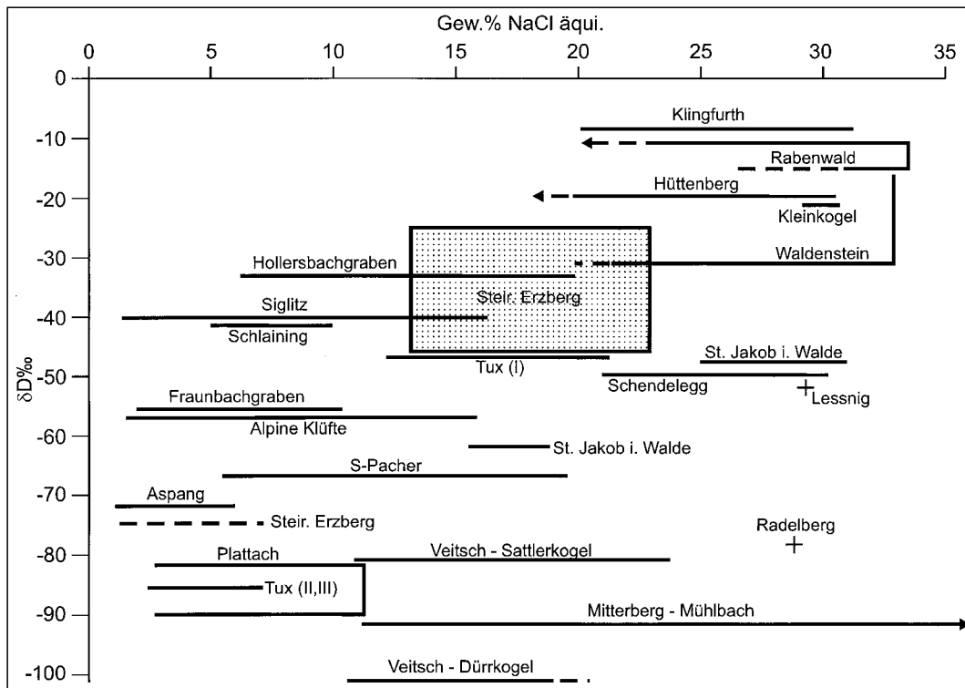
Abb. 391. \Delta\alpha\gamma\rho\epsilon\alpha\mu \delta D vs Gew.-% NaCl äquiv.
