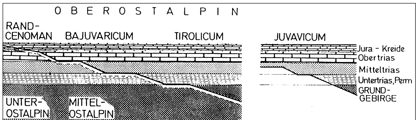
Abb. 105. Der schräge Basalzuschchnitt der ostalpinen Decken bewirkt die tektonische Amputation des Zentralalpinen Mesozoikums und dessen unterschiedliche stratigraphische Reichweite. Aus GENSER, J. & NEUBAUER, F. (1990).
