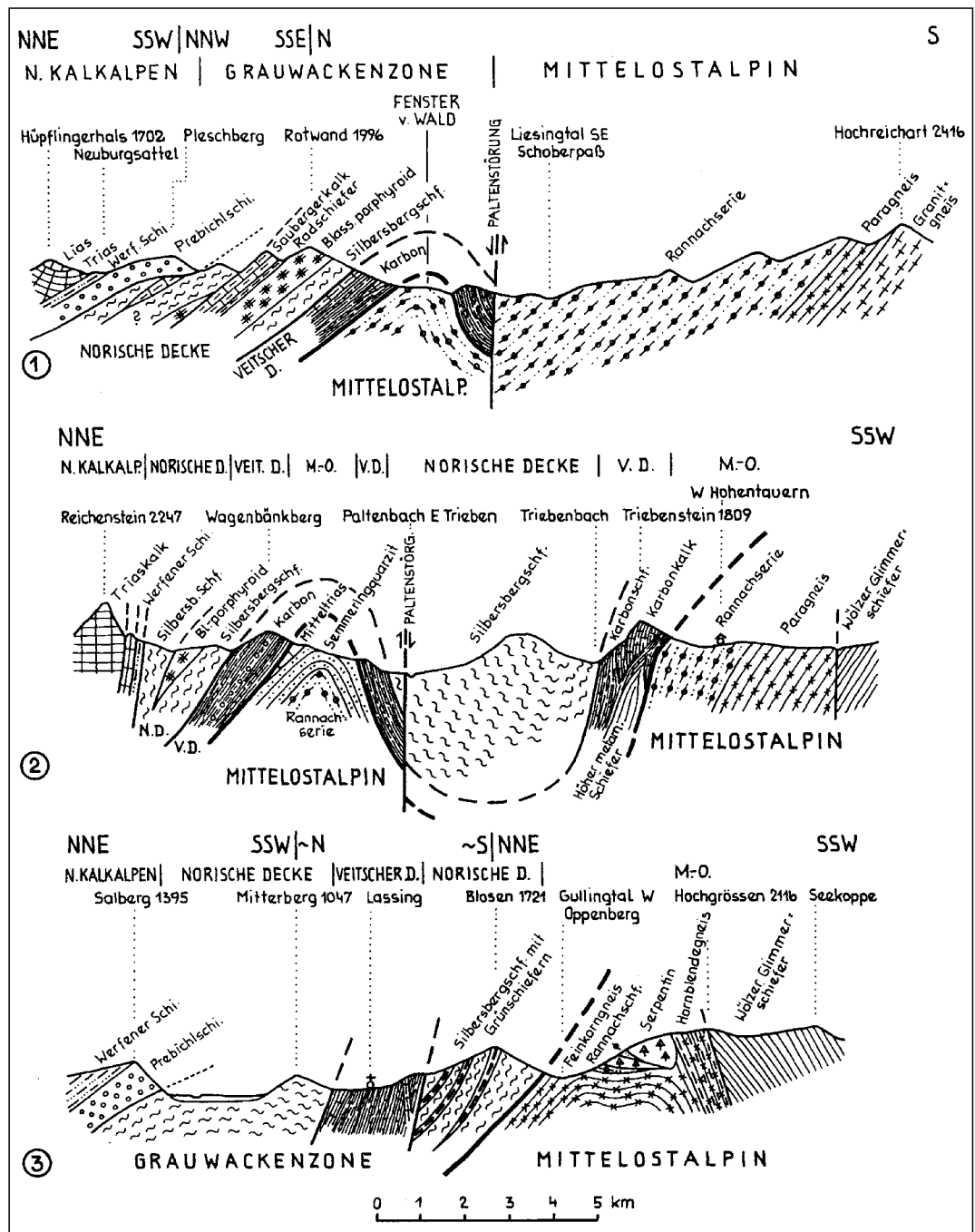
Abb. 152. Profile durch die westlichen Teile der steirischen Grauwackenzone. Teilweise dürften die Silberberg-Schiefer mit der Silberberg-Decke korrelierbar sein. Aus TOLLMANN, A. (1977a).
