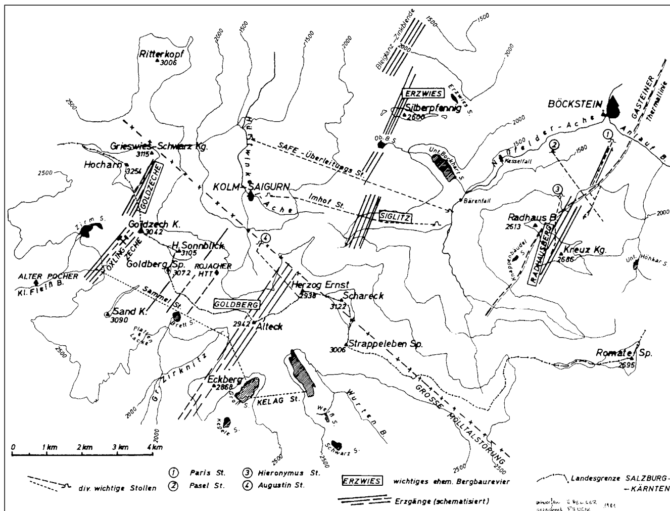
Abb. 248. Position der Tauerngoldgänge in den ehemaligen Gasteiner, Rauriser und Oberkärntner Bergbaurevieren. Nach WELSER, H. (1981).
