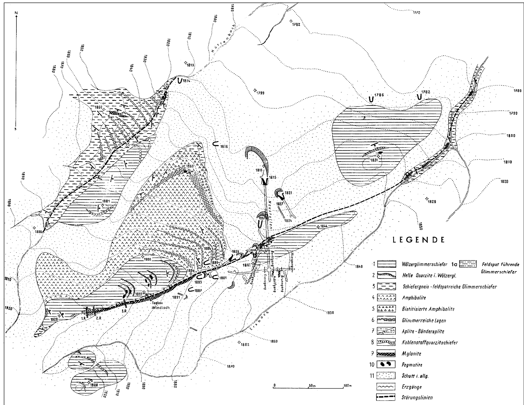
Abb. 269. Detailkarte des Erzgebietes im Plattenkar. Nach THURNER, A. (1955).
