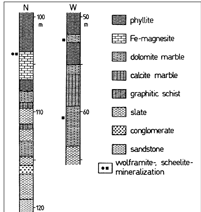
Abb. 292. Schematisches Profil durch das Wolframervorkommen Mallnock. Aus NEINAVAI, H. et al. (1989).
