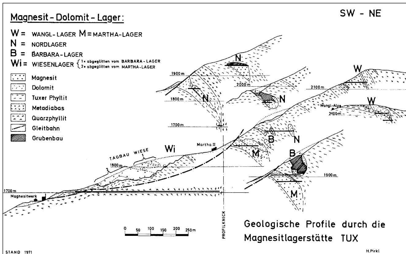
Abb. 274. Profil durch die Magnesit-Scheelitlagerstätte Tux. Nach H. PIRKL (1976; unveröffentlicht).
