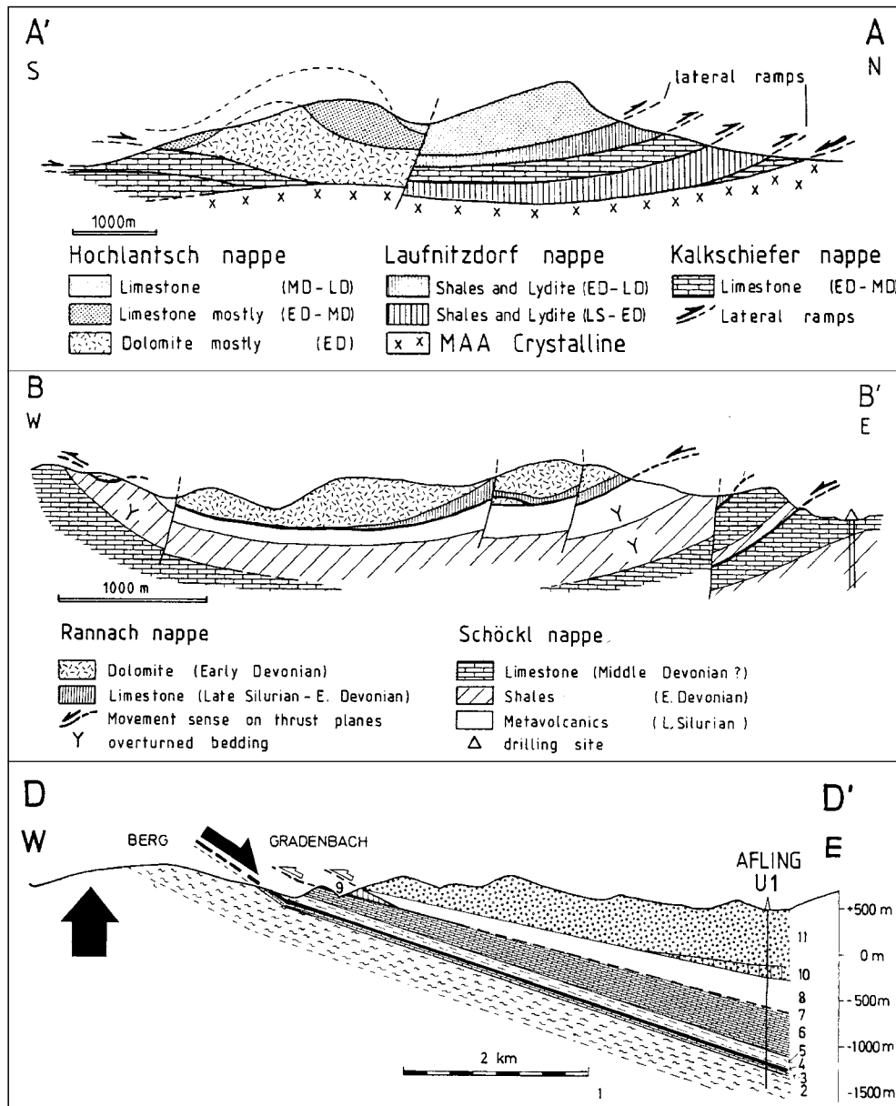
Abb. 158. Profilschnitte durch das Grazer Paläozoikum und die auflagernde Kainacher Gosau. Profil D-D': 1-3 = mittelostalpinisches Kristallin, 4 = duktile Abschiebung, 6-9 = Paläozoikum von Graz (9 = Kalkschiefer Einheit), 10-11 = Kainacher Gosau. Lage der Profile in Abb. 155. Aus FRITZ, H. et al. (1981).
