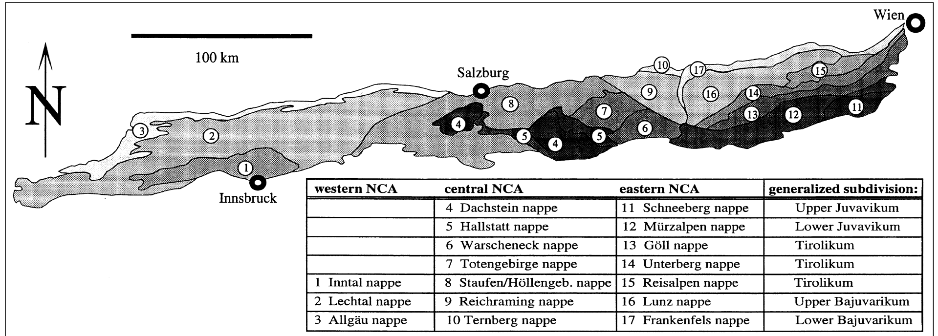
Abb. 180. Deckensysteme der Kalkalpen. Nach LINZER, H.-G. et al. (1995).
