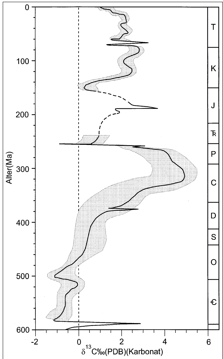
Abb. 359. Zeitabhängigkeit der Kohlenstoff-Isotopenzusammensetzung mariner Karbonate. Nach HOLSER, W.T. et al. (1995).
