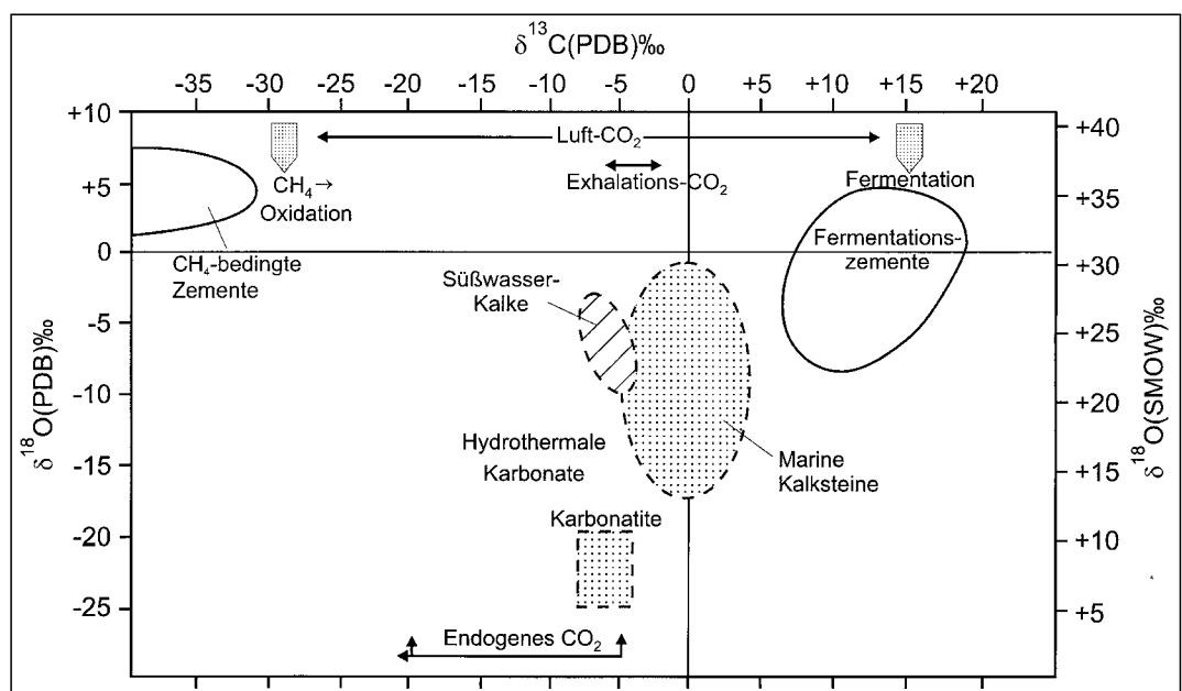
Abb. 361. Generelles Diagramm \delta^{13}C vs. \delta^{18}O . Gegenüberstellung der Kohlenstoff-Isotopenzusammensetzung des exogenen CO_2 und der biogenen Fraktionierung der Kohlenstoffisotope durch Fermentationsprozesse.
