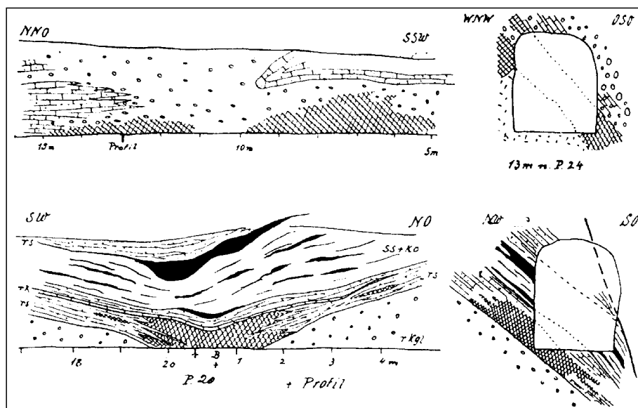
Abb. 334. Ulmbilder aus dem Revier Prefing – Sonnberg, Mittelbau II, 637 m über N.N. Oben: Übergang roter dünnplattiger Kalkschiefer und von Bauxit (Bw/Bo) in rote Konglomerate, z.T. mit bauxitischem Bindemittel. Dazu ein Querschnitt: Geröll-Lage im Bauxit, in der Firne. Unten: Übergang von Bauxit (Bw) in rote Kalkschiefer. Überlagert von Kohlschiefern mit Steinkohlenschmitzen. Dazu ein Querprofil. Nach HABERFELNER, F. (1951).
