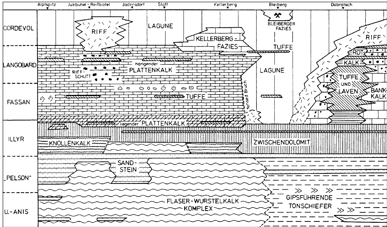
Abb. 195. Die Faziesentwicklung in der Mittel- und tiefen Obertrias im westlichen Drauzug. Aus TOLLMANN, A. (1977a) nach BECHSTÄDT, T. et al. (1976).
