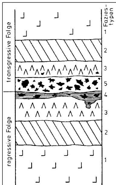
Abb. 196. Standardzyklus im Wettersteinkalk der Bleiberger Fazies. 1 = heller subtidaler Megalodontenkalk; 2 = intertidaler Flaserkalk mit Fenstergefügen; 3 = inter- bis supratidale Dolomite mit Fenstergefügen und Trockenrissen; 4 = grau-grüne mergelige Dolomite („grüne Mergel“); 5 = schwarze Breccien. Aus BECHSTÄDT, T. (1975a).
