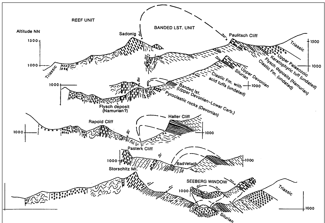
Abb. 207. Querprofile durch die Südkarawanken im Seeberggebiet südlich Eisenkappel. Aus BAUER, F.K. & SCHÖNLAUB, H.P. (1980b) nach ROLSER, J. & TESSEN- SOHN, F. (1974).
