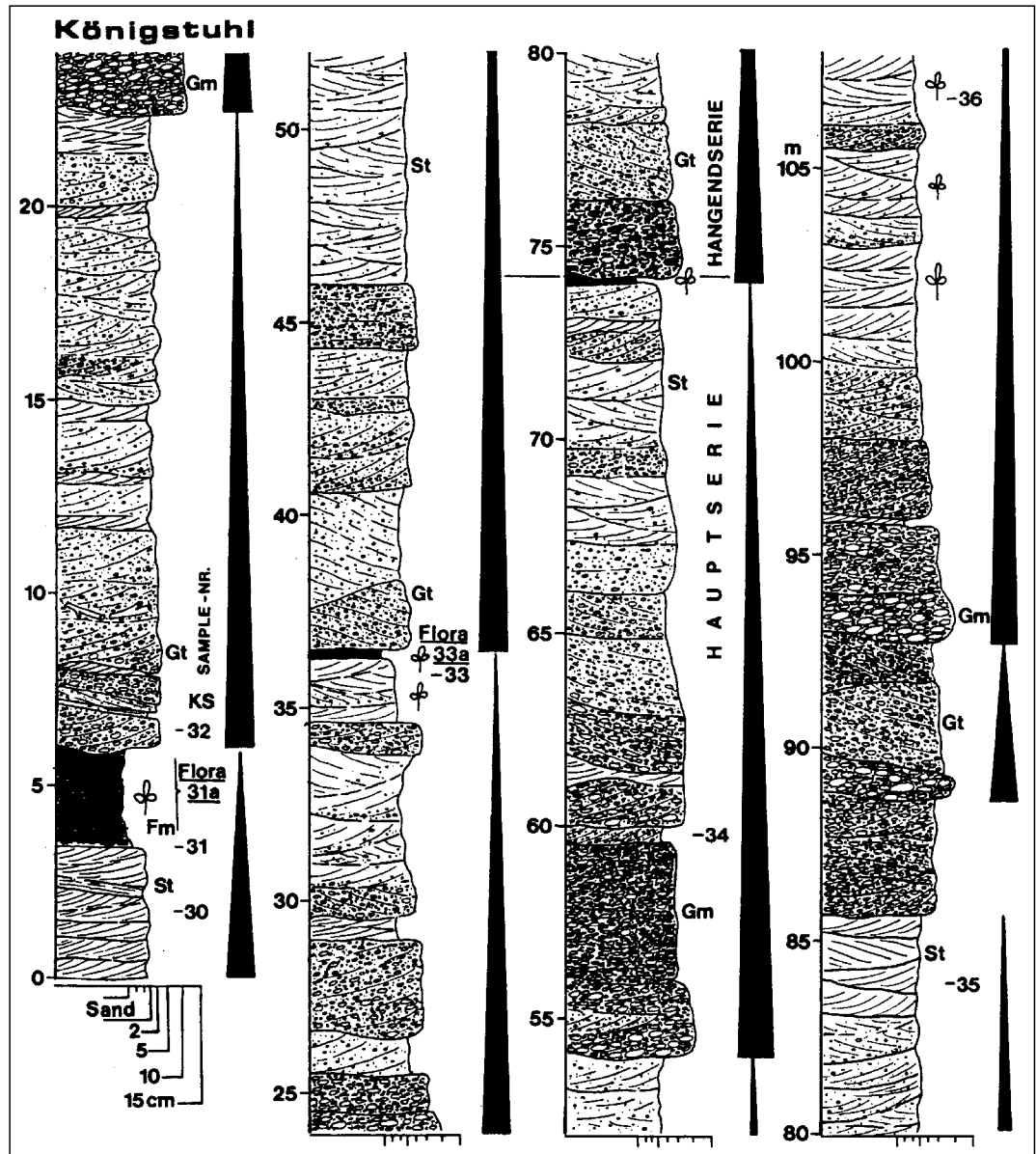
Abb. 90. Beispiel oberkarboner in- tramontaner Beckenfü- llungen (Stangnock Fm. der Gurktaler Decke). Gm = massige Konglo- merate; Gt = kreuzge- schichtete Konglomerate; St = Sandsteine; Fm = Overbank Sedimente. AUS KRAINER, K. (1989, 1993)
