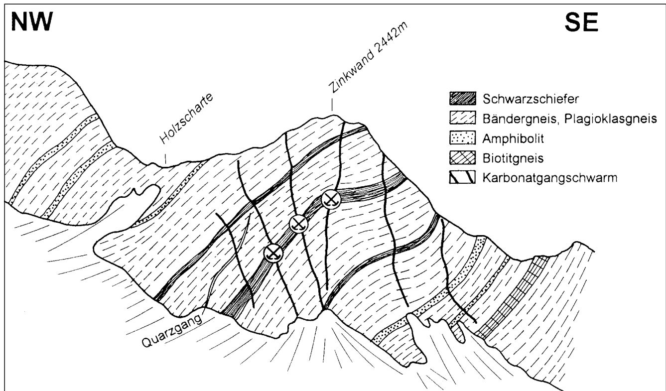
Abb. 263. Profilsansicht der SW-Seite der Zinkwand, Schladminger Tauern, mit Lokation der Haupteinbaue. Nach SCHEDL, A. (1981); Zeichnung: H.P. STEYERER.
