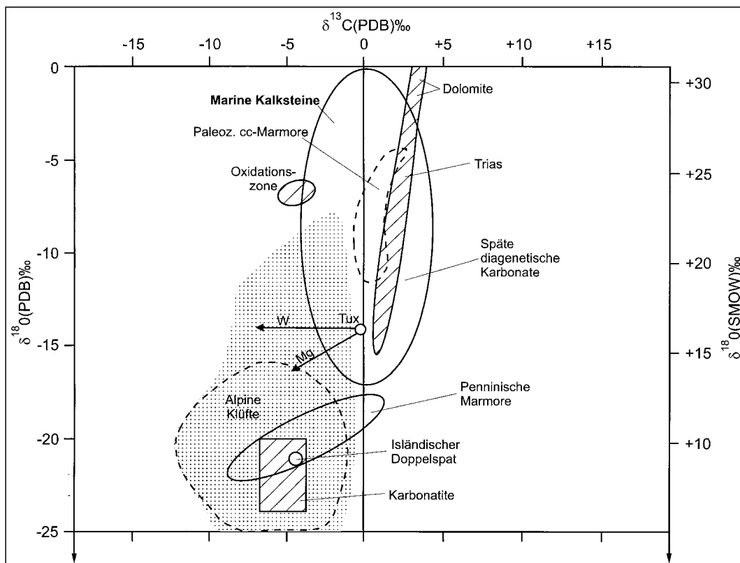
Abb. 362. \delta^{13}\text{C} vs. \delta^{18}\text{O} -Diagramm vorzugsweise von Calciten und Kalksteinen aus den Ostalpen. Die Karbonate der scheel- itführenden Magnesit- Lagerstätte Tux-Laners- bach unterscheiden sich isotonenmäßig nach den Paragenesen mit Scheelit (W) und mit Magnesit (Mg).
