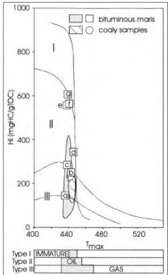
Abb. 337. Wasserstoffindizes (HI) gegen T_{max} -Werte (Pyrolysetemperatur, bei der ein Maximum an KW neu gebildet wird) für kohlige Proben und Bitumenmergelproben aus der Kainacher Gosau. Kreise und Quadrate kennzeichnen Kerogenkonzentrate. Das organische Material besteht aus Mischungen von allochthonem terrigenem Kerogen Typ III und autochthonem wasserstoffreichem Material (Kerogen Typ I). Es befindet sich im Bereich des Ölfensters. Verändert nach SACHSENHOFER, R.F. (1995).
