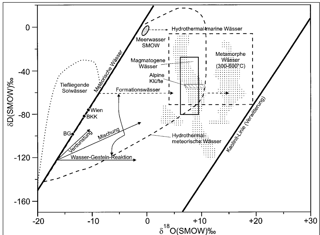
Abb. 358. \delta^{18}\text{O} - vs. \delta^{13}\text{D} -Diagramm (modifiziert nach SHE- PARD, S.M., 1977 und an- deren Quellen) mit der Eintragung der \delta\text{D} - und \delta^{18}\text{O} -Werte von in den Ostalpen mineralisieren- den Fluiden. Auf der Linie der Nieder- schlagswässer BKK = Bad Kleinkirchheim und BG = Bad Gastein.
