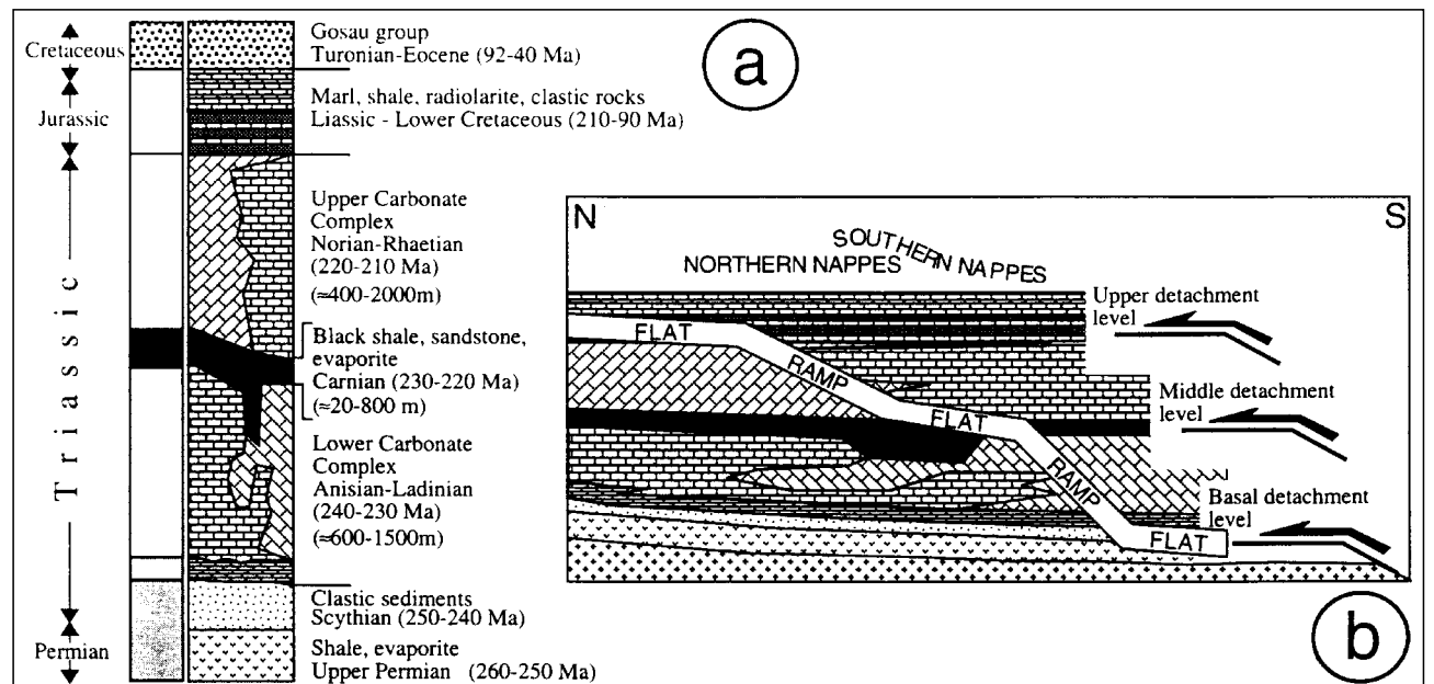
Abb. 181. a) Generalisierte Schichtsäule der Kalkalpen. b) „Ramp-flat“-Geometrie: die tektonisch tieferen und nördlicheren Decken wurden in höheren stratigraphischen Niveaus abgesichert als die tektonisch höheren und südlicheren Bereichen entstammenden Decken. Nach LINZER, H.-G. et al. (1995).
