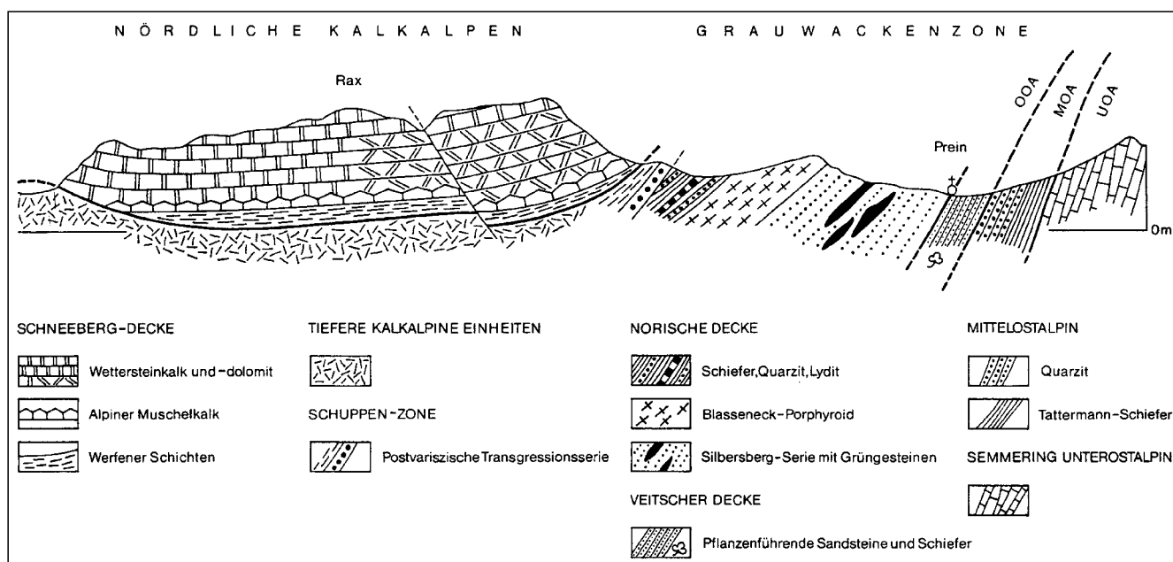
Abb. 154. Querprofil durch die östliche Grauwackenzone im Bereich der Veitsch (die Silbersberg-Serie entspricht der Silbersberg-Decke). Aus SCHÖNLAUB, H.P. (1979).
