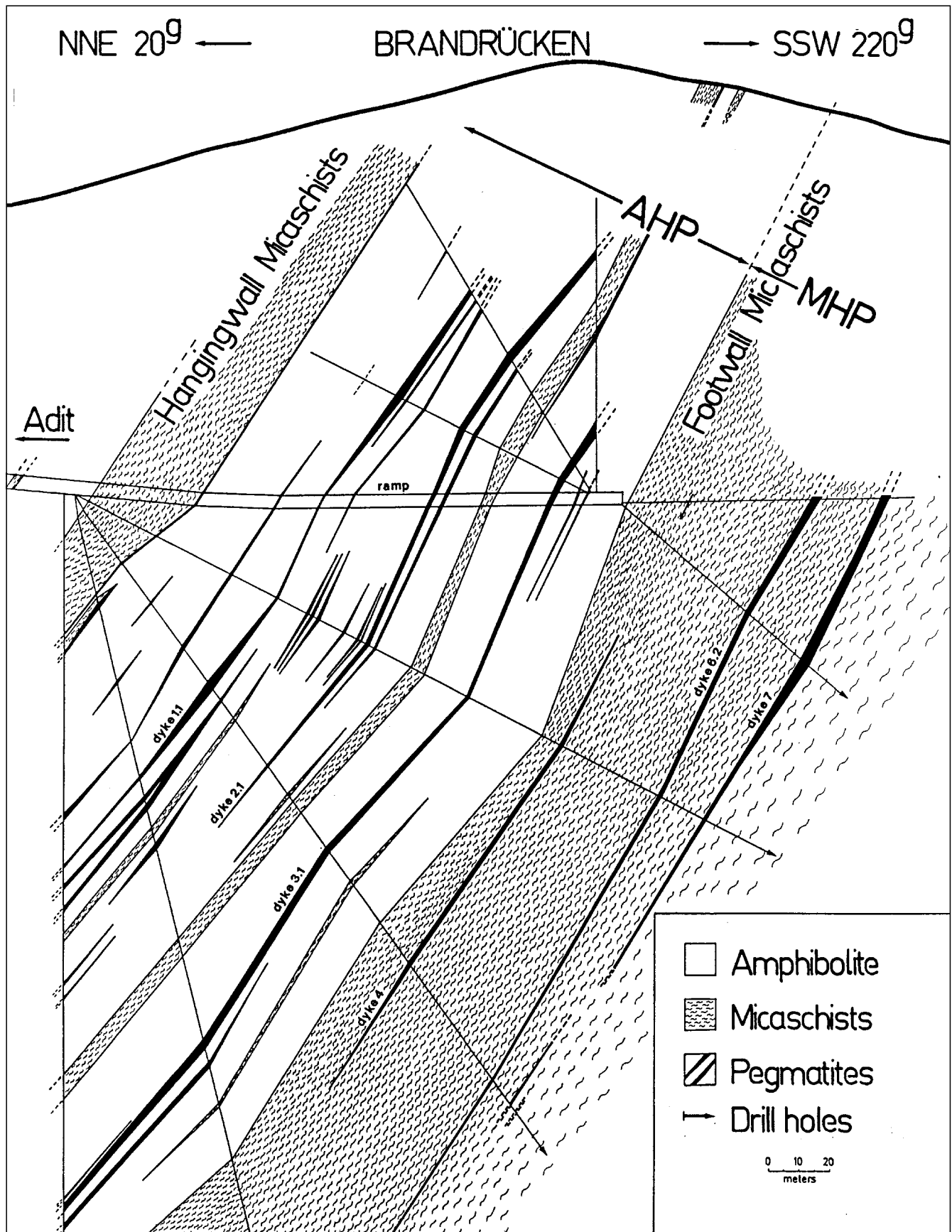
Abb. 268. Geologisches Profil durch die Spodumenlagerstätte am Brandrücken. Nach R. Göb.
