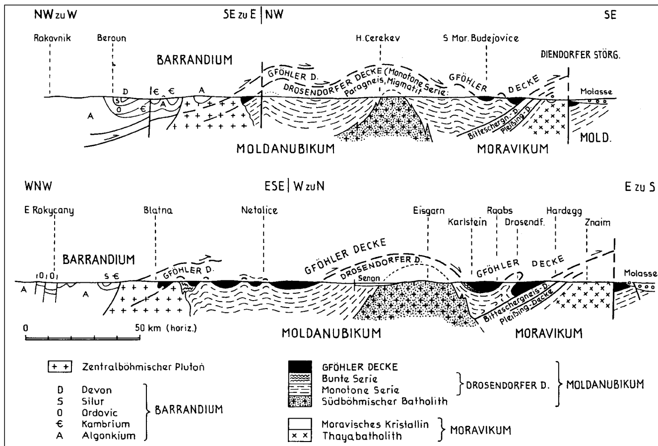
Abb. 14. Profile zum Deckenbau in der Böhmischen Masse. Aus TOLLMANN, A. (1985).
