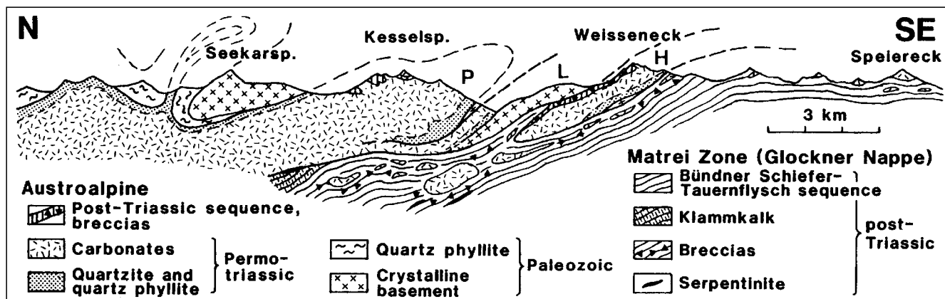
Abb. 103. ▲ ▲ ▲ Profil durch den Tauern-NE-Rand (Matreier Zone) und die Radstädter Tauern nördlich von St. Michael/Lungau. H = Hochfeind-Decke; L = Lantschfeld-Decke; P = Pleising-Decke. Nach TOLLMANN, A. (1964) und FRISCH, W. et al. (1987).
