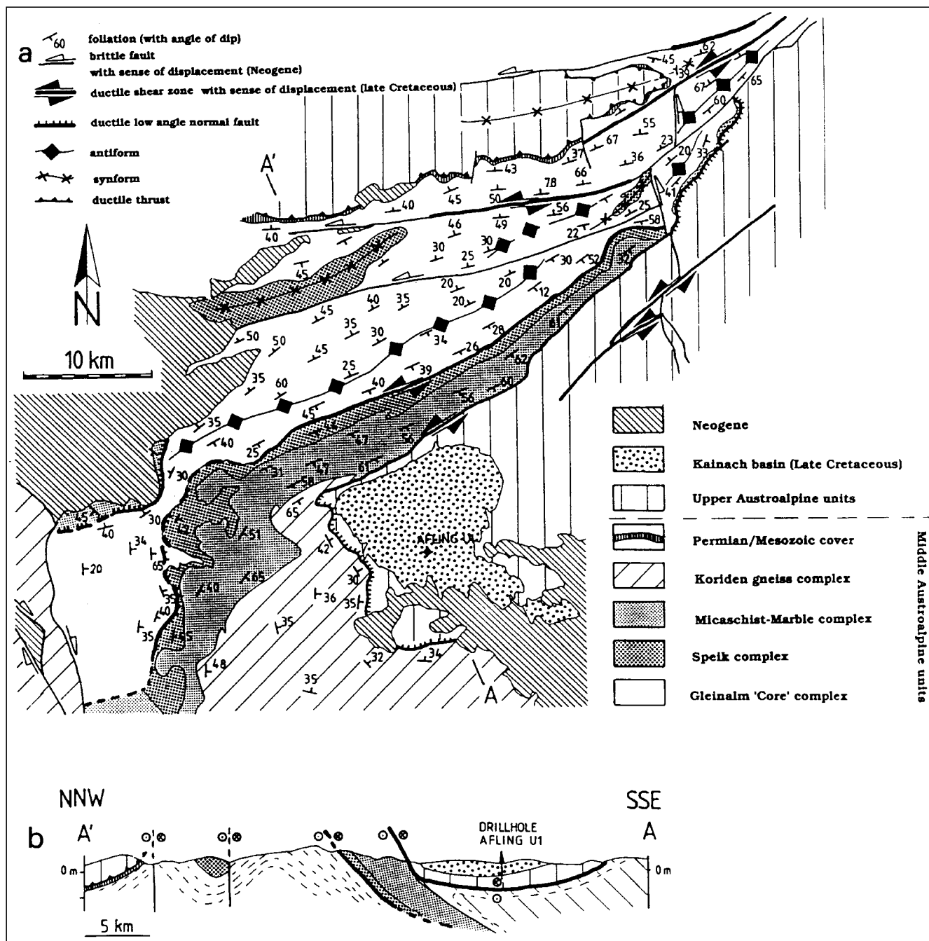
Abb. 131. Tektonische Karte und Profil durch den Gleinalm-Kern mit einer ENE-streichenden Antiklinalstruktur, randlichen steilstehenden duktilen Scherzonen und flachen Abschiebungen. Aus NEUBAUER, F. et al. (1995).
