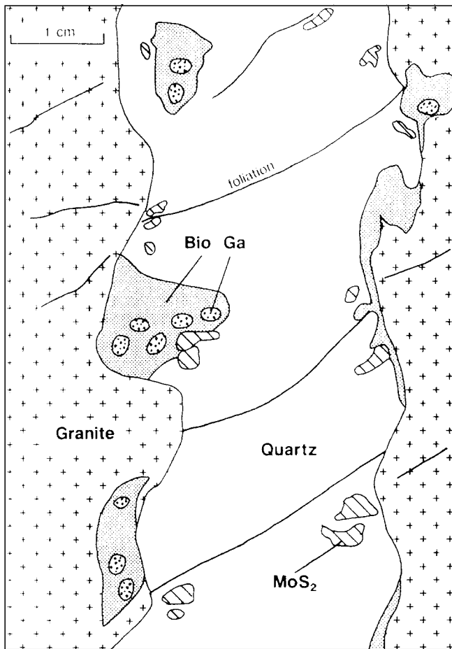
Abb. 240. Schematische Darstellung eines Molybdänit-führenden Quarzganges der Alpeiner Scharte. AUS MELCHER, F. et al. (1996).
