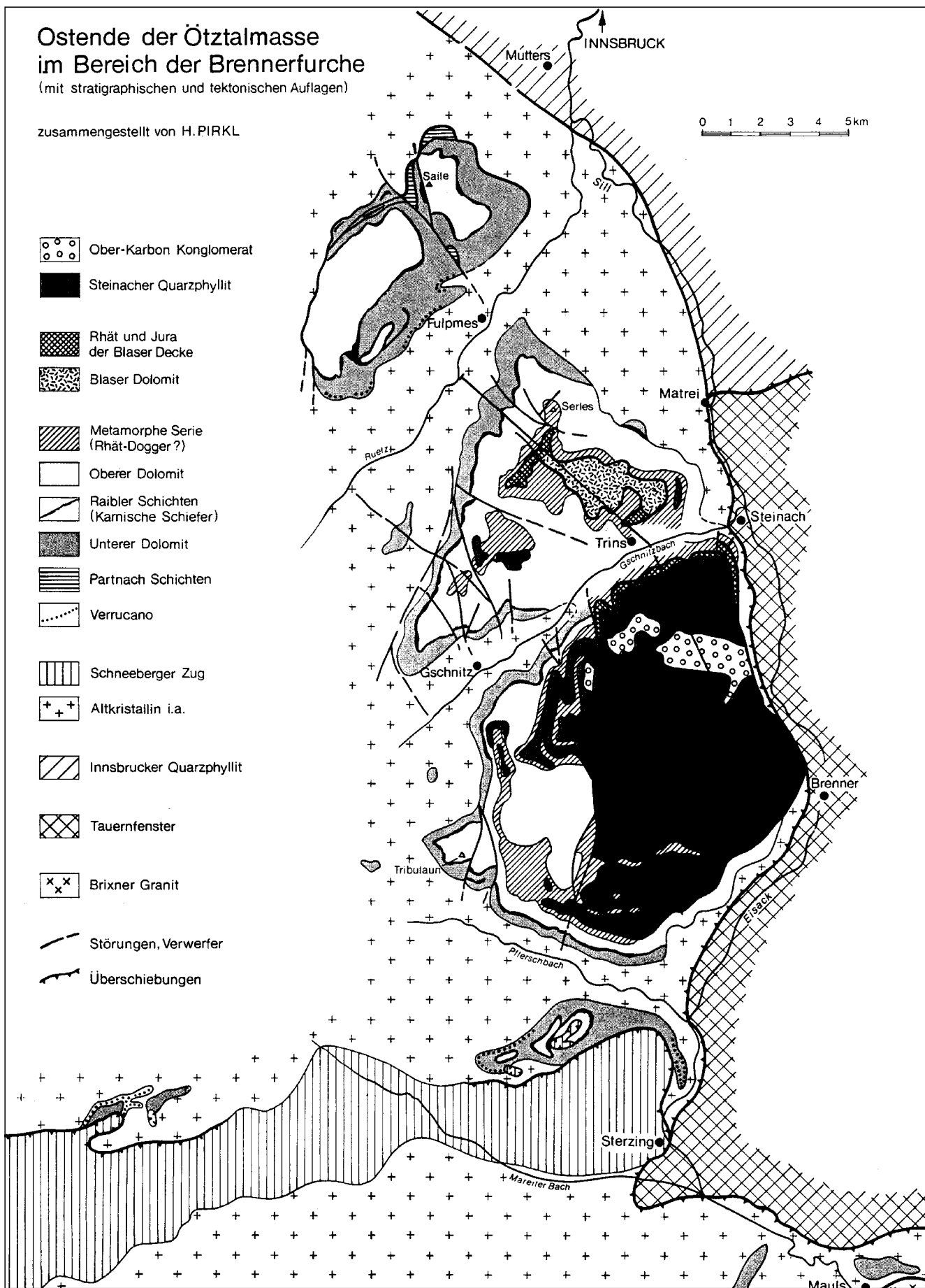
Abb. 108. Zentralalpines Mesozoikum, Blaser und Steinacher Decke am Ostrand des Ötztal-Kristallins (aus PIRKL, H., 1980).
