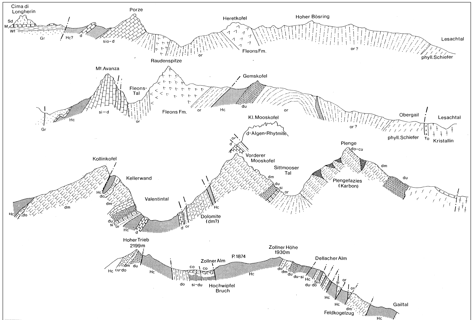
Abb. 205. Profilserie durch die westlichen und zentralen Karnischen Alpen. Aus BAUER, F.K. & SCHÖNLAUB, H.P. (1980a).
