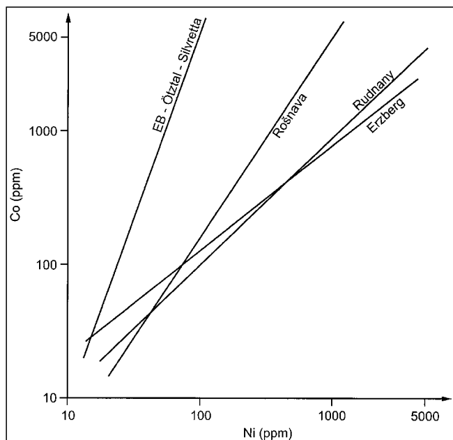
Abb. 344. Regressionsgeraden der Ni/Co-Korrelation von Pyriten des Steirischen Erzberges (MALEKGASEMI, F., 1979), aus den Sideritlagerstätten Rosnava und Rudnany in den Westkarpaten (CAMEL, B. & JARKOVSKY, J., 1970) und den Cu-Fe-Vererzungen des Erzbezirkes Stubai-Ötztal (VAUTAR, F., 1988).
