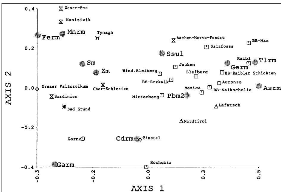
Abb. 393. Korrespondenzanalyse unter Verwendung von Datenmaterial (Konzentrationen von As, Cd, Ga, Ge, Mn und Tl) in Sphaleriten und Isotopenparametern ( \delta^{34}\text{S} ) in allen Sulfiden (Sm), im Sphalerit (Zm) und Sulfaten (Ssul) sowie dem Isotopenmilieuwert des Bleis (Pbm2) unter Einbeziehung von 26 Lagerstätten. Aus SCHROLL, E. et al. (1996).
