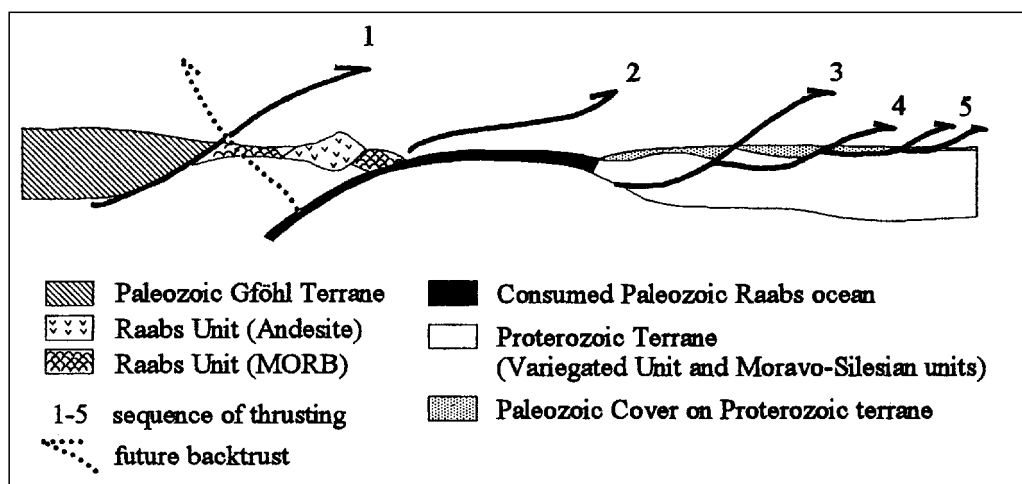
Abb. 15. Tektonisches Schema der südöstlichen Böhmischen Masse mit Schließung eines ozeanischen Bereichs (Raabs Ozean) und einem nach NE in seichtere Krustenniveaus propagierenden Deckensystem.
