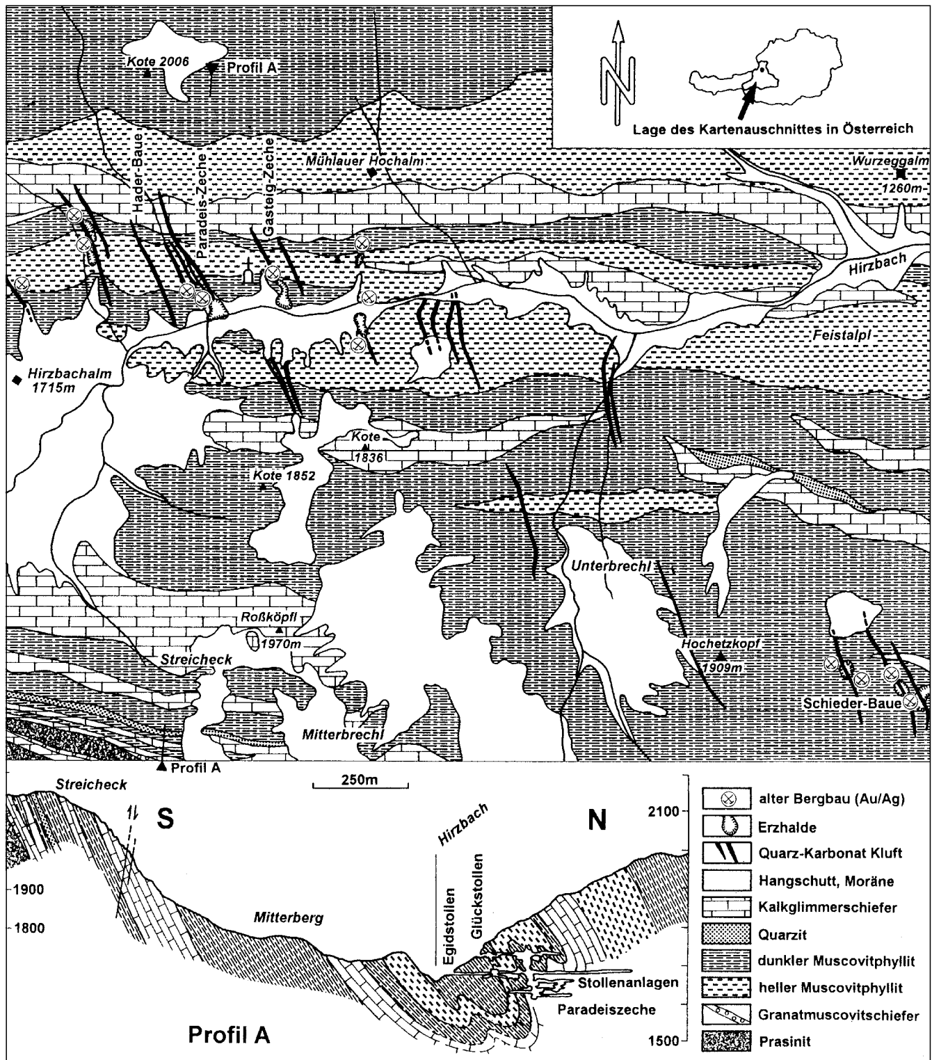
Abb. 252. Geologie tektonisch kontrollierter Gold- Silber-Lagerstätten des Hirzbach-Schiedalpe-Kloben-Typus in der Bündnerschiefer-Formation. Nach BRANDMAIER, P., (1989); Zeichnung: H.P. STEYERER.
