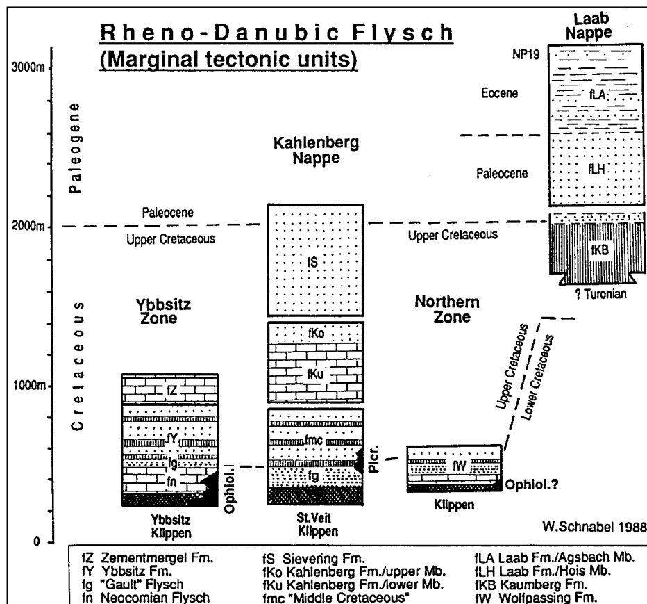
Abb. 59. Die Schichtfolgen der Ybbsitzer Zone, der Kahlenberg- und Laaber Decke in der östlichen Flyschzone. Aus SCHNABEL, W.G. (1992).
