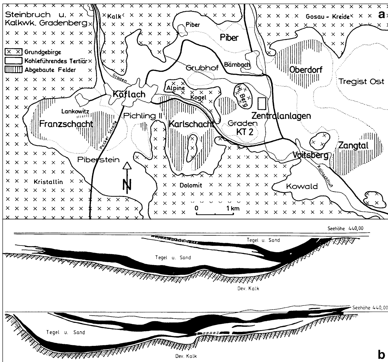
Abb. 229. Köflach-Voitsberger Braunkohlenbezirk. a) Verbreitung der Kohlenmulden. b) schematisches geologisches Profil durch die Lagerstätte Karlschacht. AUS WEBER, L. & WEISS, A. (1983).
