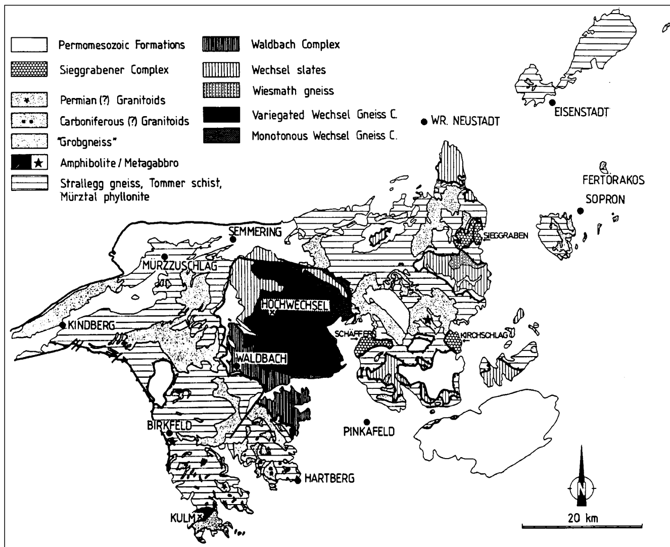
Abb. 119. Verbreitung unterostalpinischer Einheiten am Alpenostrand. Lediglich der Siegrabener Komplex wird dem „Mittelostalpin“ angegliedert. Aus NEUBAUER, F. & FRISCH, W. (1993).
