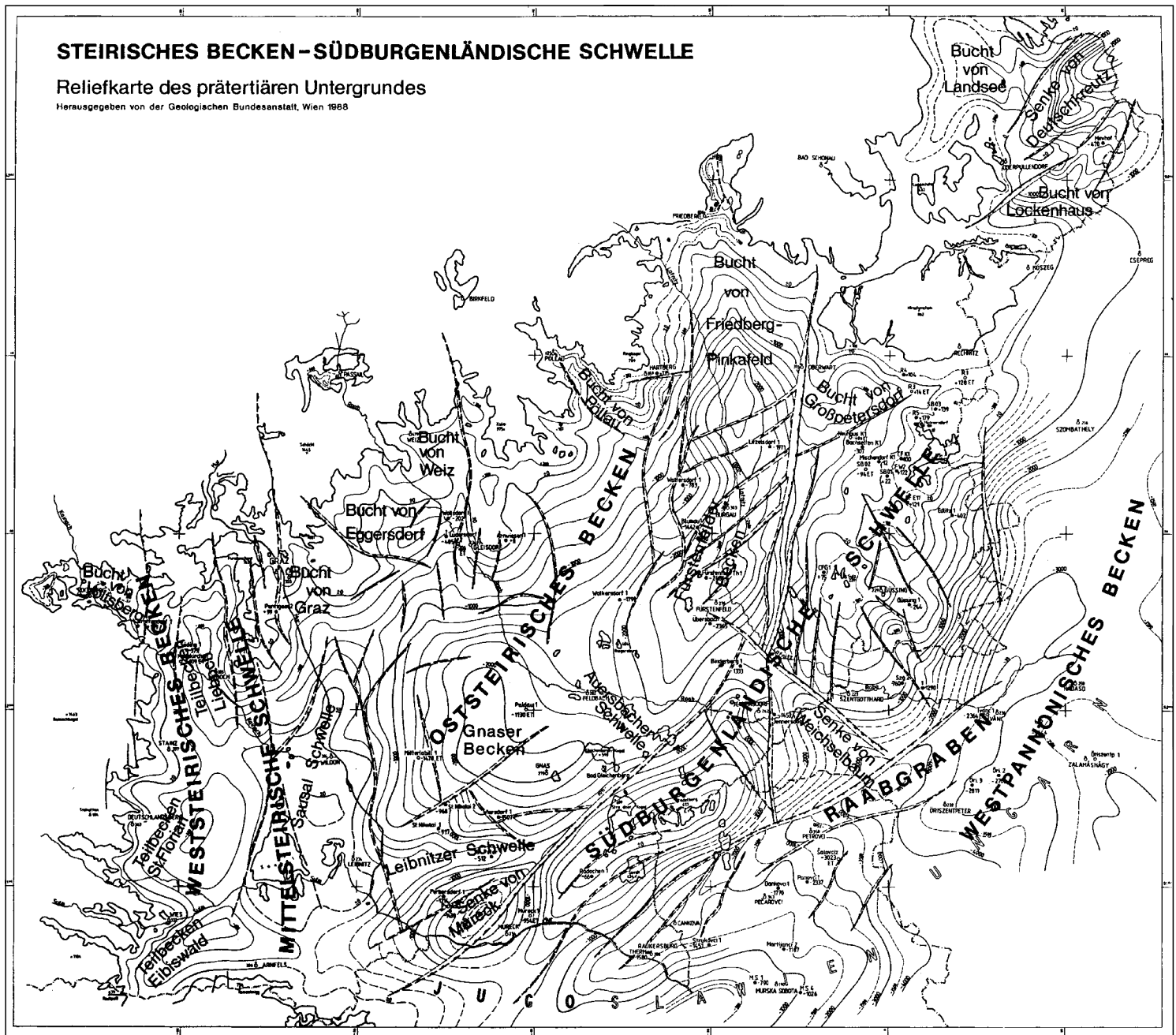
Abb. 40. Reliefkarte des prä-tertiären Untergrundes im Steirischen Becken. Neue Aufschlußergebnisse zeigen einen wesentlich größeren Tiefgang für das Gnaser Becken als in der Abbildung dargestellt. Aus KRÖLL, A. et al. (1988).
