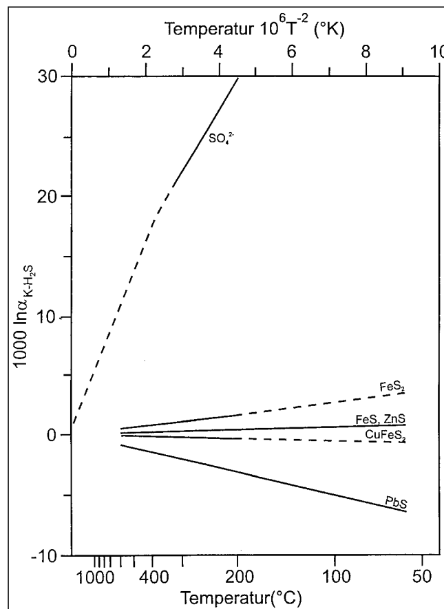
Abb. 369. Fraktionierung der Schwefelisotopen von Sulfat und einigen wichtigen Sulfid Erzmineralen. Modifiziert nach RYE, R.O. & OHMOTO, H. (1974).
