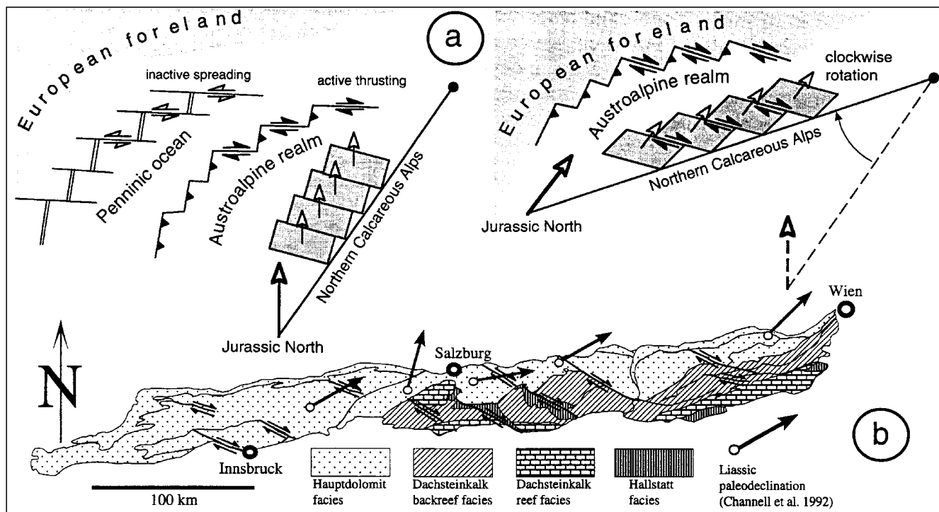
Abb. 185. a) Geometrisches Modell zur Bildung wichtiger Strukturelemente in den Kalkalpen. b) Die Zerlegung der Kalkalpen in Blöcke bedingt durch die schräge Konvergenz wird teilweise durch die Versetzung der Großfaziesbereiche nachgezeichnet. Nach LINZER, H.-G. et al. (1995).
