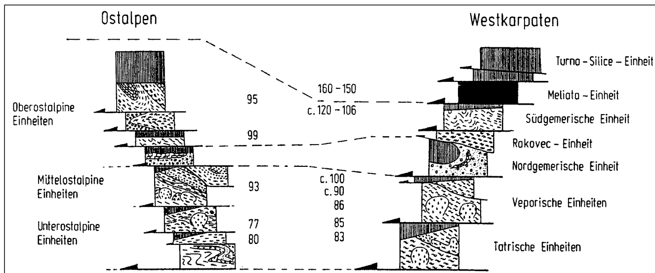
Abb. 22. Tektonostratigraphisches Schema der ostalpinen Einheiten im Vergleich mit jenen der Westkarpaten und ^{40}\text{Ar}/^{39}\text{Ar} -Alter (in Ma) aus Hellglimmern längs der Deckenbahnen, die Hinweise auf das Überschiebungsalter geben (NEUBAUER, F., 1994).
