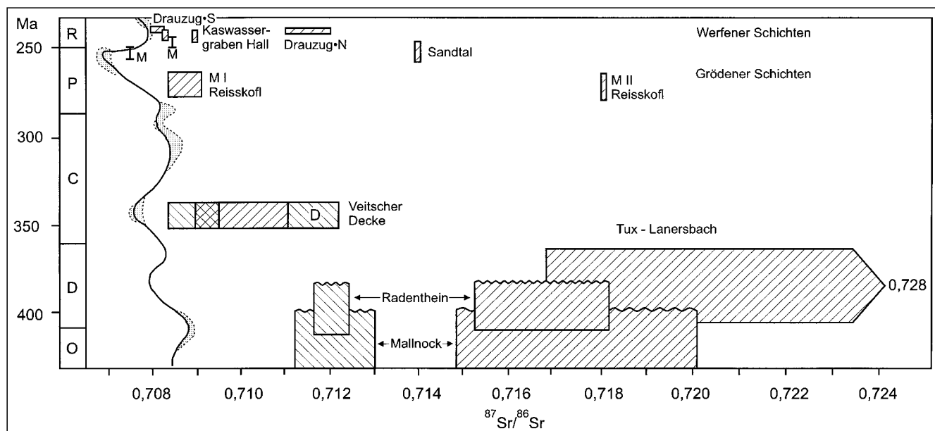
Abb. 374. Strontiumisotopen-Verteilung in Magnesitvorkommen. Rechtsschraffur = Magnesit; Linksschraffur = Dolomit. Modifiziert und ergänzt nach FRIMMEL, H. & NIEDERMAYR, G. (1991).
