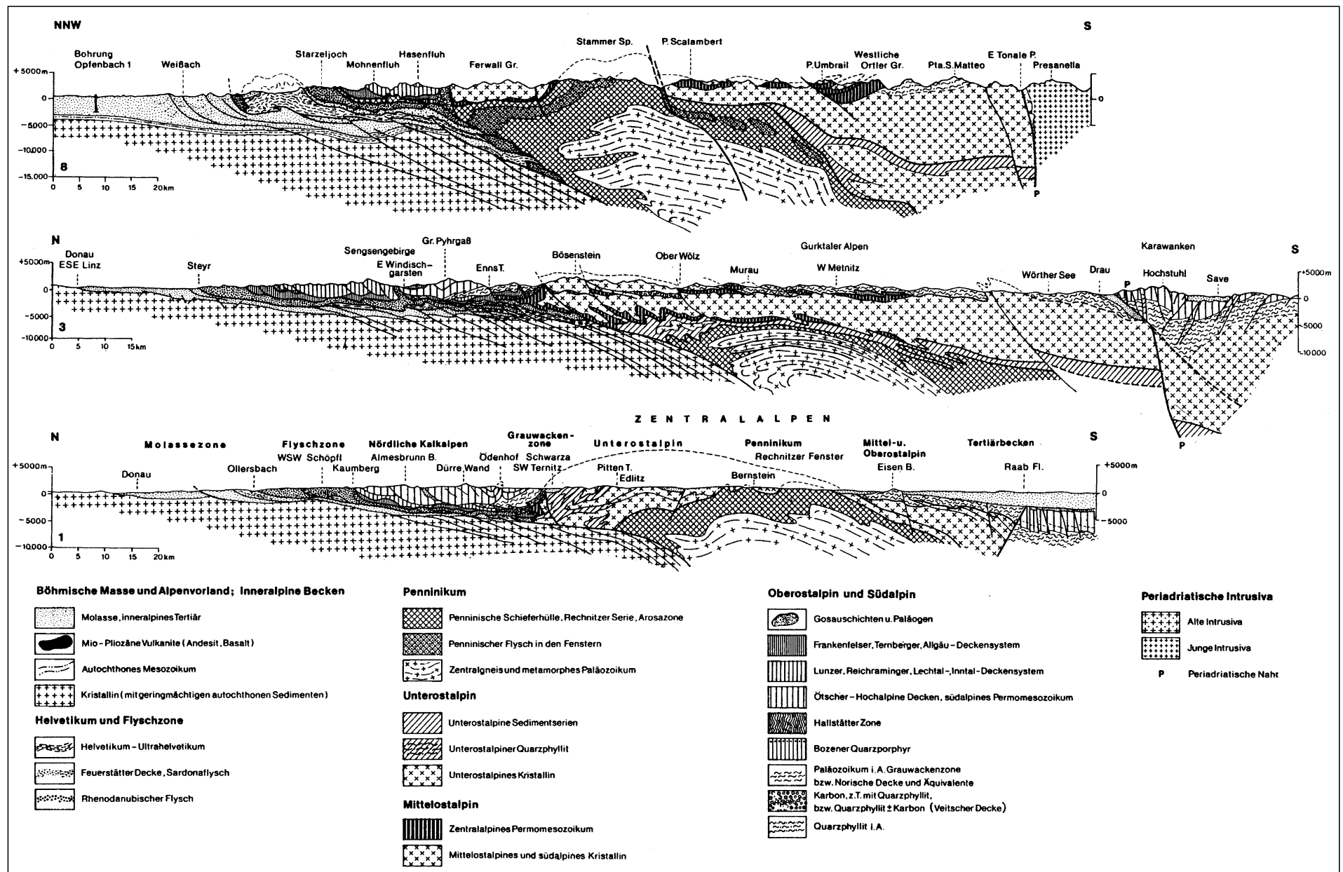
Abb. 24. Nord-Süd-Profile durch die Ostalpen (nach PREY, S., 1980a). Von oben nach unten: Profil 1 = durch das Engadiner Fenster; Profil 2 = Steyr – Wörther See; Profil 3 = durch den Alpenostrand und die Rechnitzer Fenstergruppe.
