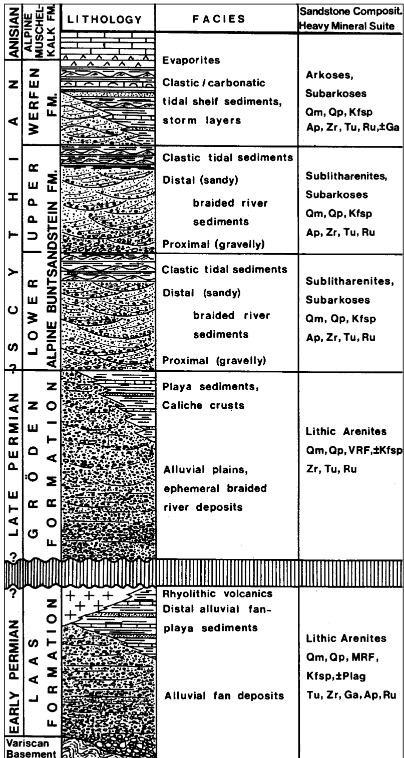
Abb. 193. Lithostratigraphisches Profil und Fazies der permoskythischen Basisentwicklung des Drauzuges. Sandsteinzusammensetzung: Qm = monokristalliner Quarz; Qp = polykristalliner Quarz; Kfsp = Kalifeldspat; Plag = Plagioklas; VRF = Vulkanitkomponenten; MRF = metamorphe Gesteinskomponenten; Schwerminerale: Ap = Apatit; Ru = Rutil; Ga = Granat; Tu = Turmalin; Zr = Zirkon. Aus KRAINER, K. (1993).
