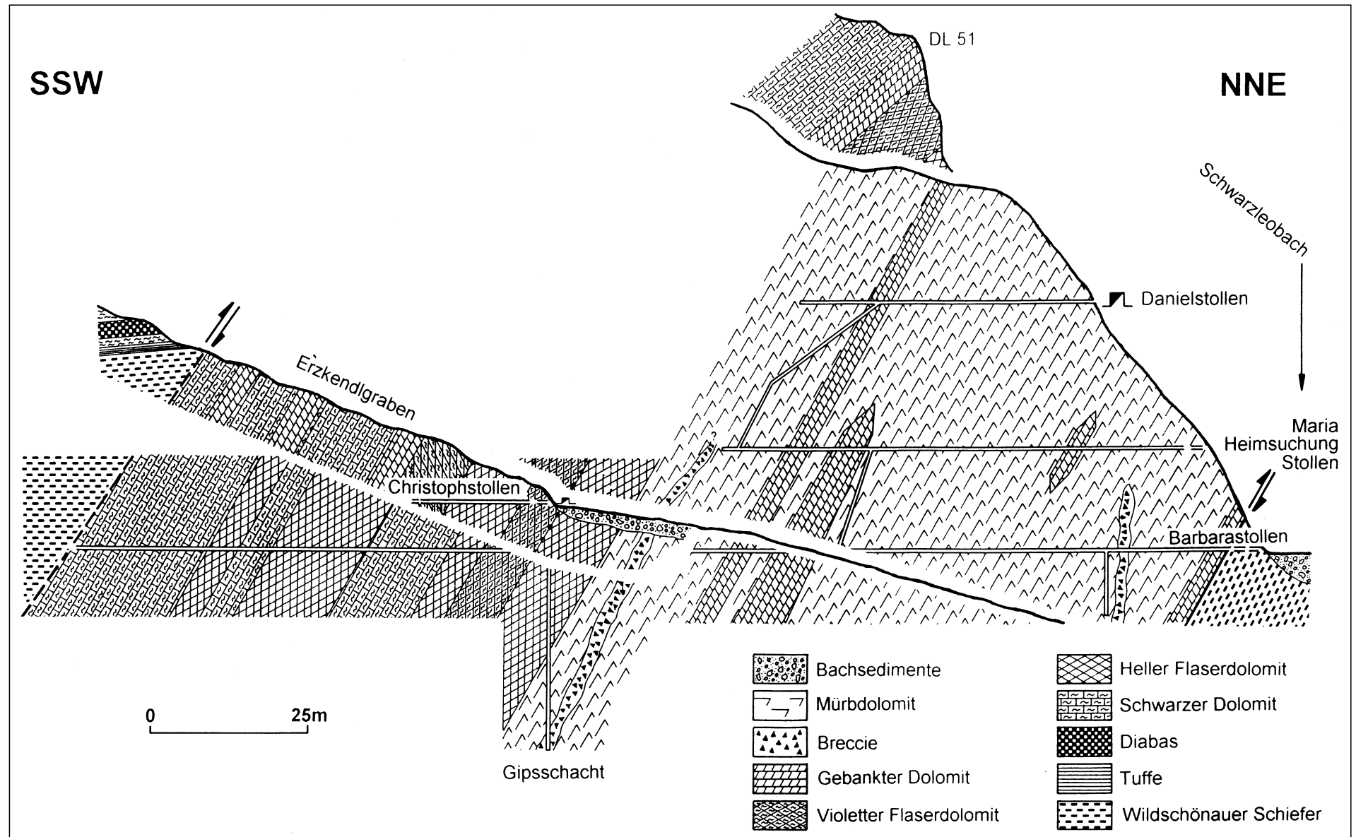
Abb. 279. Revier Schwarzeleo (Leogang, Salzburg): geologisches Idealprofil. Nach LENGAUER, C. (1989); Zeichnung: H.P. STEYRER.
