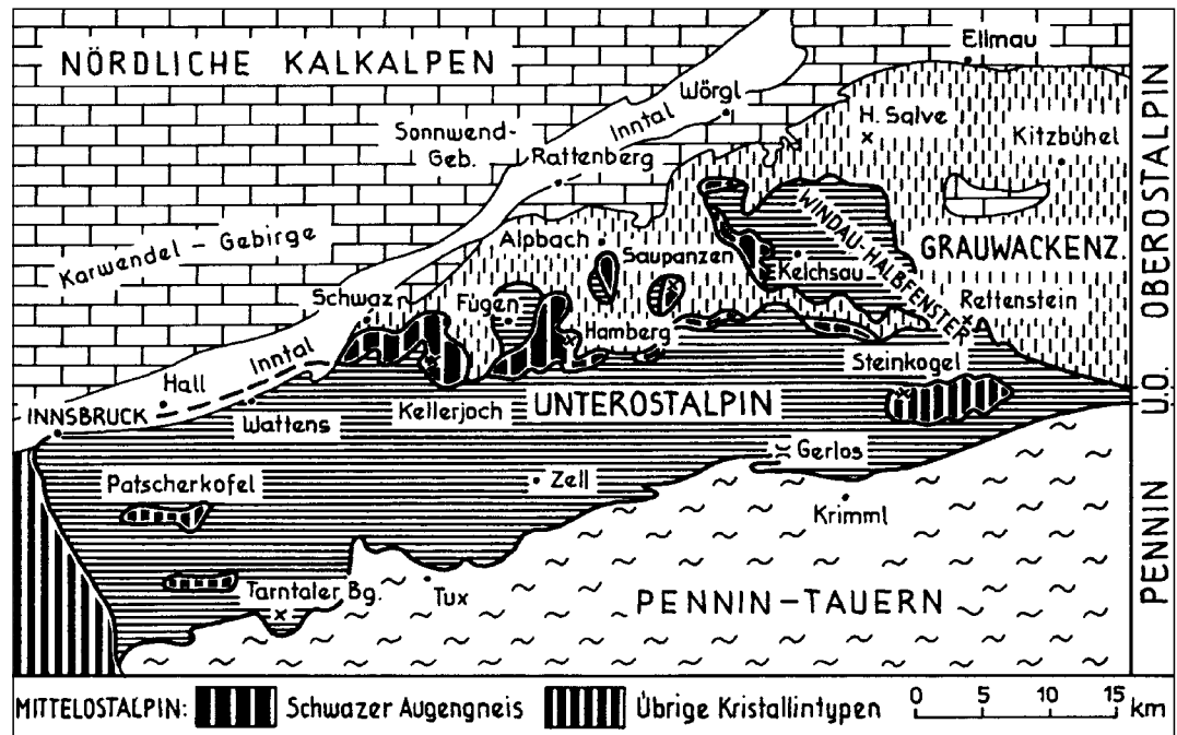
Abb. 111. Die „mittelostalpinen“ Kristallinschollen mit dem Schwarzer Augengneis und den Steinkogelschiefern zwischen Innsbrucker Quarzphyllit und Grauwackenzone. AUS TOLLMANN, A. (1977a).
