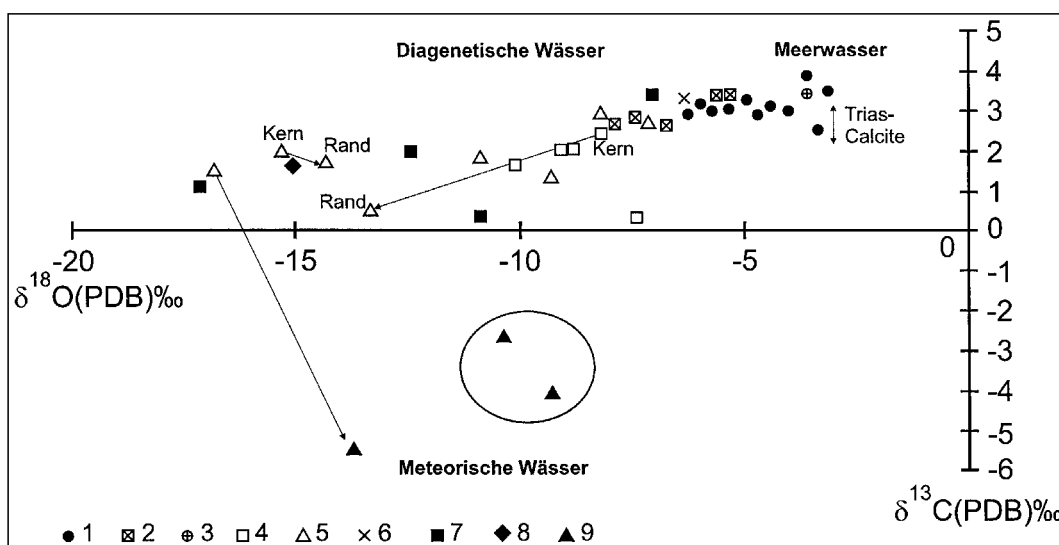
Abb. 363. Isotopenverteilung in Calciten und Dolomiten (Gesteine und Gangart) in der Blei-Zinklagerstät- te Bleiberg. 1 = Wettersteinkalk (un- vererzt und vererzt); 2 = Carditadolomit; 3 = Stro- matolith (Dolomit); 4 = Skalenoederspat; 5 = Ka- nonenspat (Posterz- Calcit); 6 = fibriger Calcit; 7 = derber Calcit; 8 = Strontianit; 9 = rhomboe- drischer Calcit (Oxi- dationszone).
