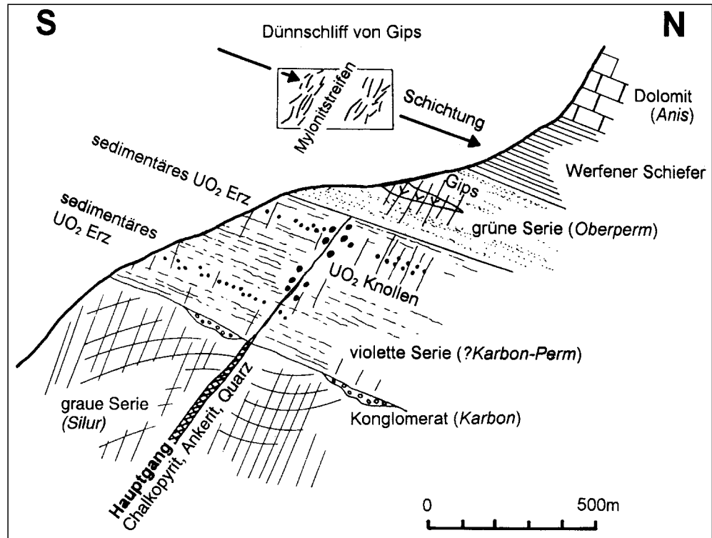
Abb. 280. Der Hauptgang der Mitterberger Kupfererzlagstätte, Schema der Schieferung und der Uranführung. Nach PETRASCHECK, W.E. (1976). Zeichnung: H.P. STEYRER.
