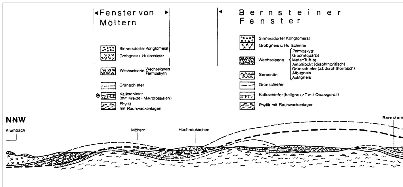
Abb. 82. Vereinfachtes Profil durch die penninischen Fenster von Möltern, Bernstein und Reintz. Nach PAHR, A. (1977) aus PAHR, A. (1980c).
