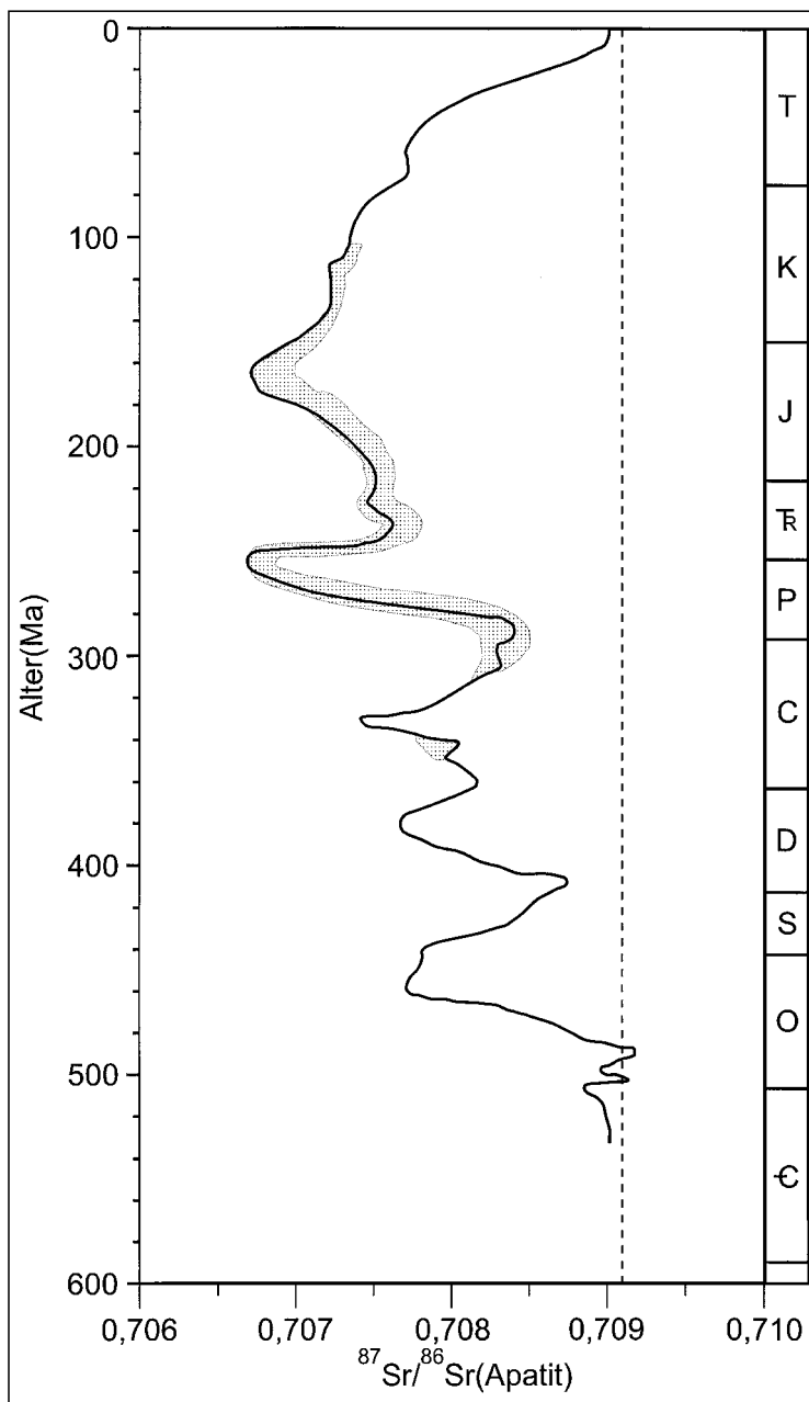
Abb. 374. Strontiumisotopen-Verteilung in Magnesitvorkommen. Rechtsschraffur = Magnesit; Linksschraffur = Dolomit. Modifiziert und ergänzt nach FRIMMEL, H. & NIEDERMAYR, G. (1991).
