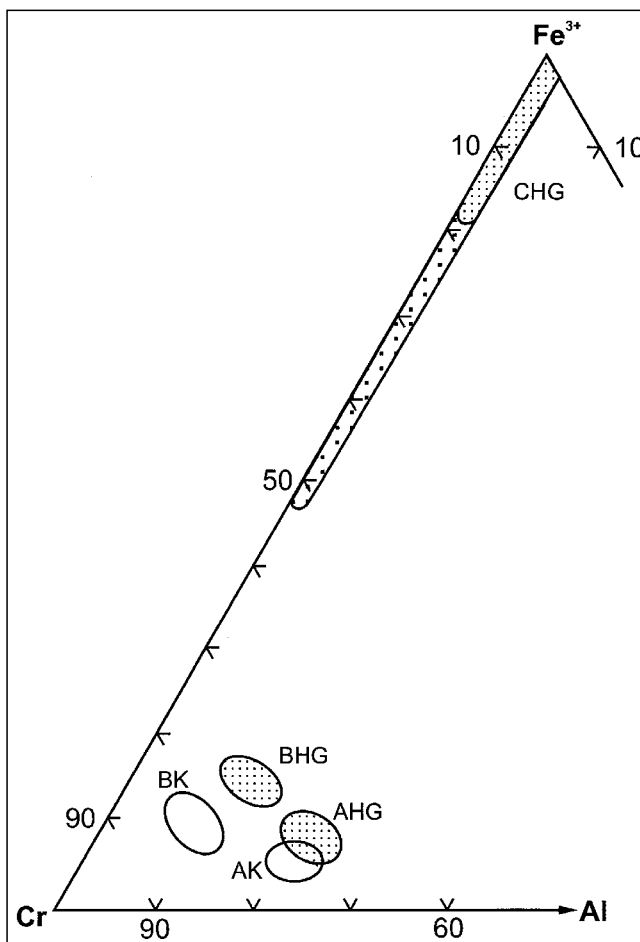
Abb. 345. Cr-Al- \text{Fe}^{3+} -Diagramm der Chromitite von Kraubath (K) und Hochgrößen (HG), differenziert nach ihrer Zonierung A (Kern), B und C. Modifiziert nach THALHAMMER, O.A.R. & STUMPF, E.F. (1988).
