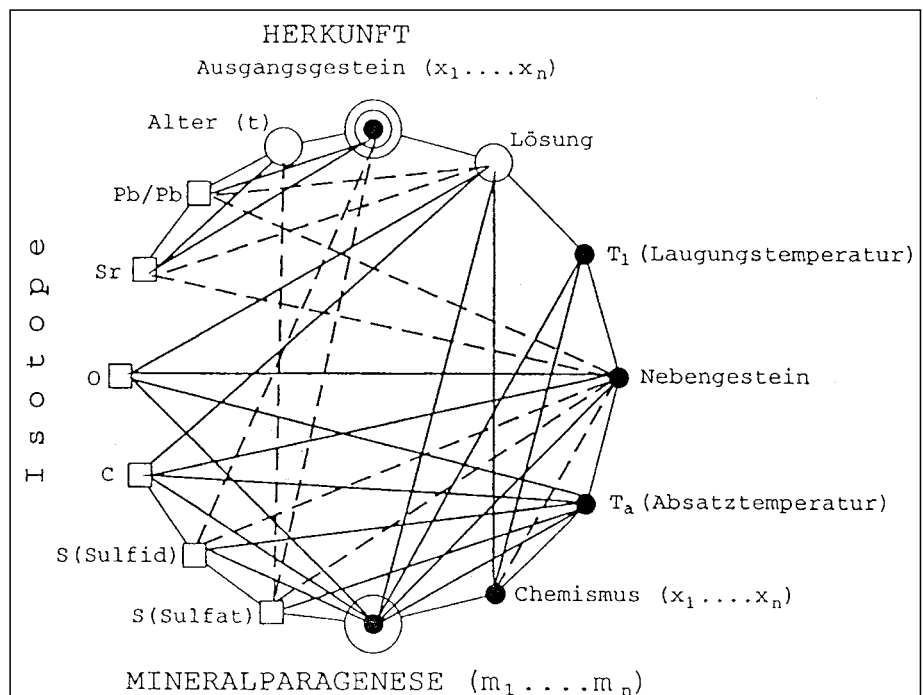
Abb. 383. Vereinfachtes vernetztes System der thermodynamischen Parameter ( T, x ) und Isotopenparameter einer hydrothermalen Erzmineralisation. Aus SCHROLL, E. et al. (1996).
